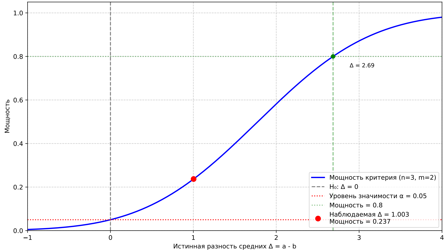
Мощность Z-критерия ( \sigma^2_x=2 , \sigma^2_y=1 , n=3 , m=2 )
