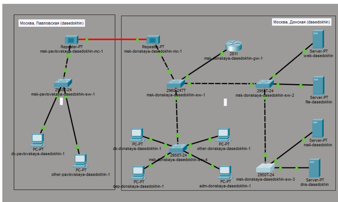
Рисунок 3.1: Размещение сервера dns и подключение его к коммутатору msk-donskaya-dasedokhin-sw-3
