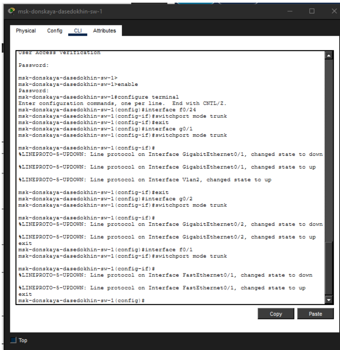
Рисунок 3.1: Настройка Trunk-порта коммутатора msk-donskaya-dasedokhin-sw-1
