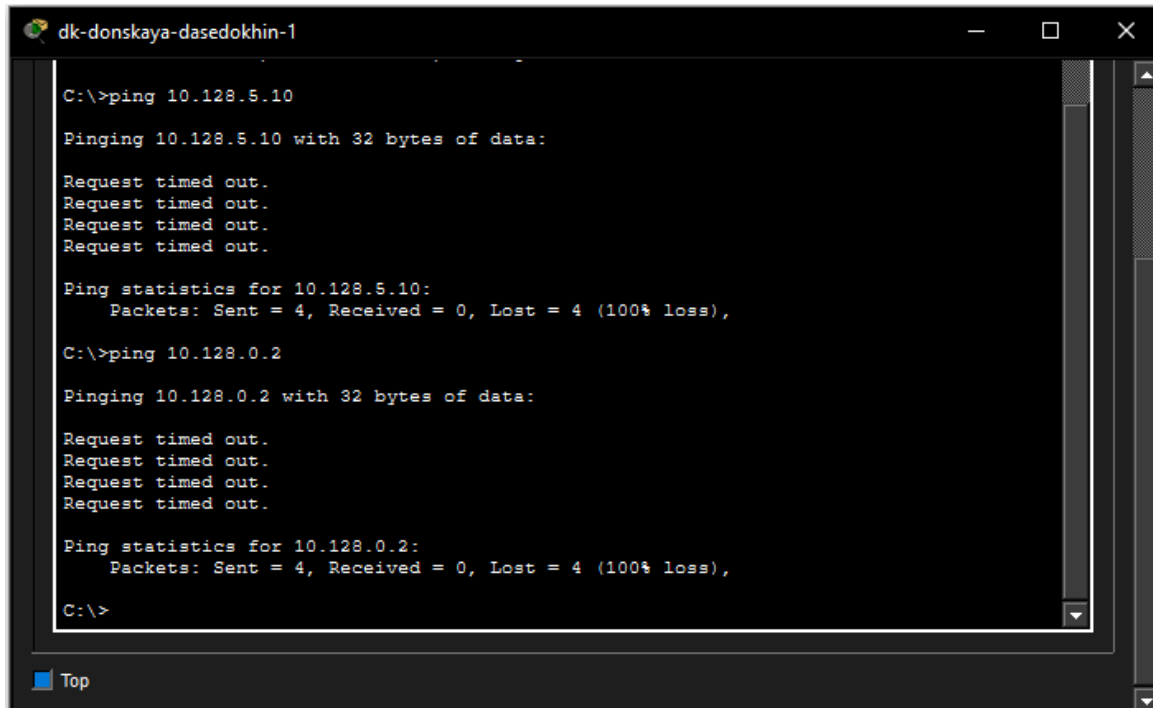
Рисунок 3.14: Пинг устройств принадлежащих разным VLAN
