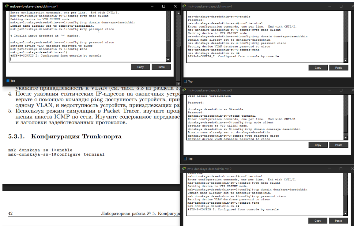
Рисунок 3.7: Наситрока msk-donskaya-sw-2 — mskdonskaya-sw-4, msk-pavlovskaya-sw-1 как VTP-клиенты
