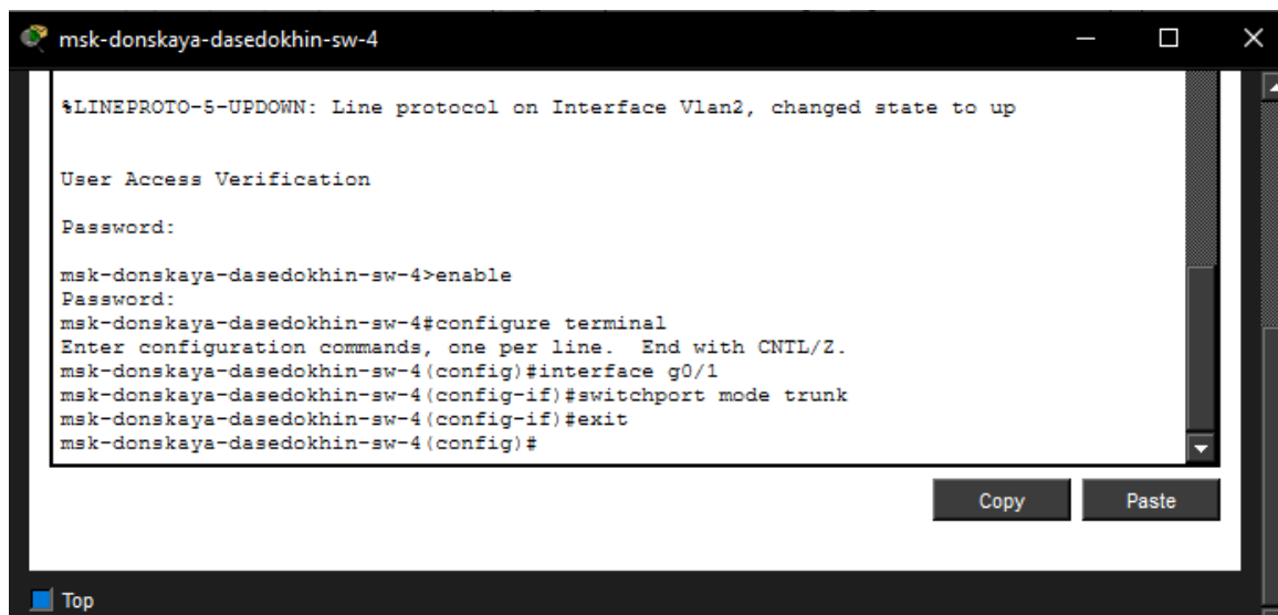
Рисунок 3.4: Настройка Trunk-порта коммутатора msk-donskaya-dasedokhin-sw-4
