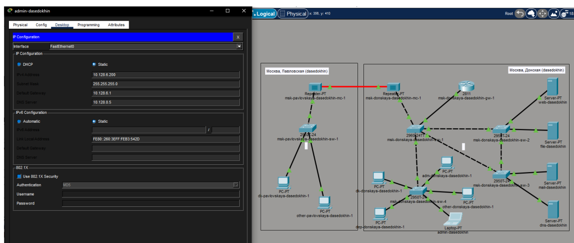
Рисунок 3.1: Размещение ноутбука администратора с именем admin-dasedokhin
