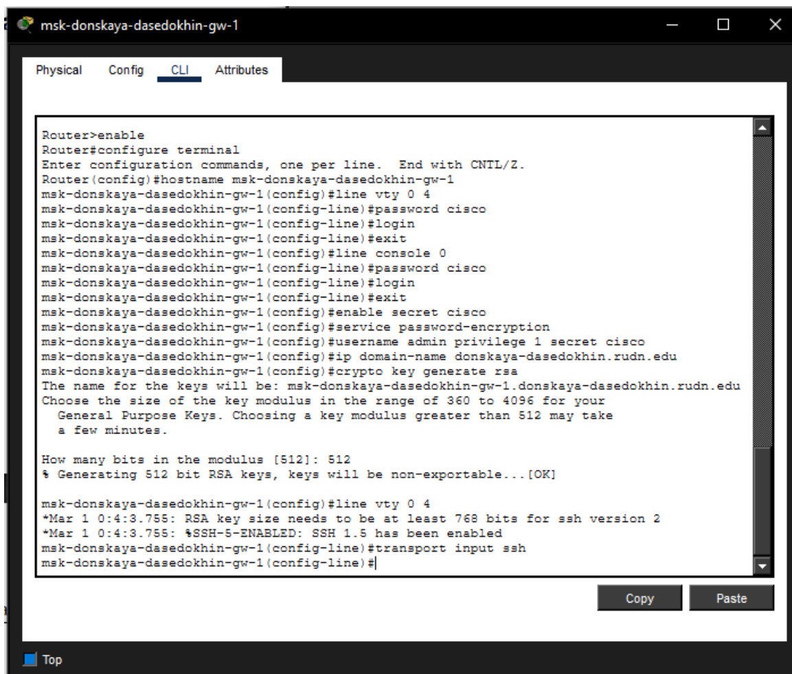
Рисунок 3.2: Настройка маршрутизатора msk-donskaya-dasedokhin-gw-1
