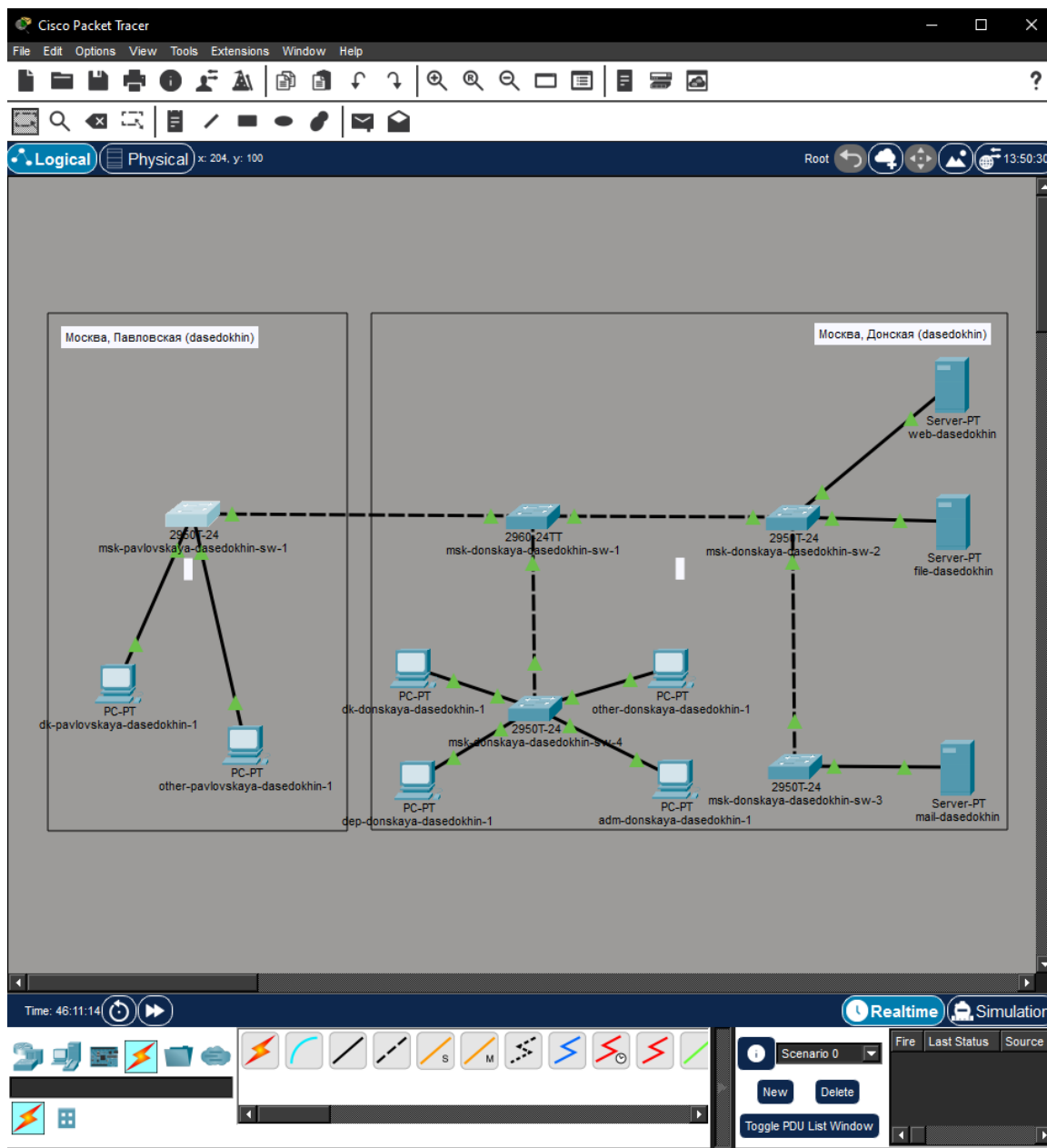
Рисунок 3.1: Размещение коммутаторов и оконечных устройств согласно схеме
