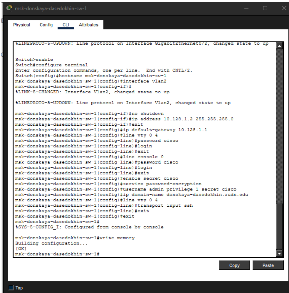
Рисунок 3.2: Настройка коммутатора msk-donskaya-dasedokhin-sw-1
