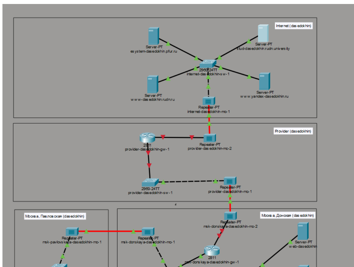
Рисунок 3.1: Воспроизведение топологии сети
