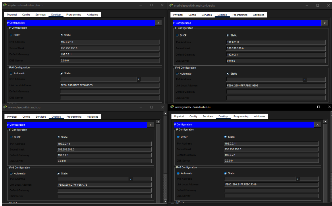
Рисунок 3.6: Конфигурация ip-адресов для серверов согласно таблице
