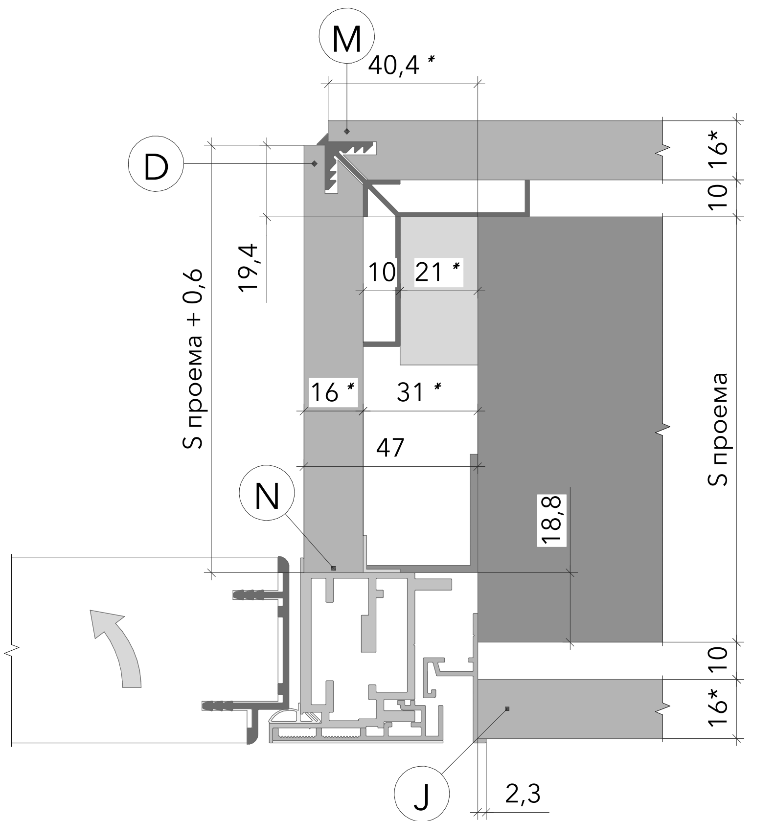
Коробка Complanar 50 Наличник Shade Открытие внутрь
