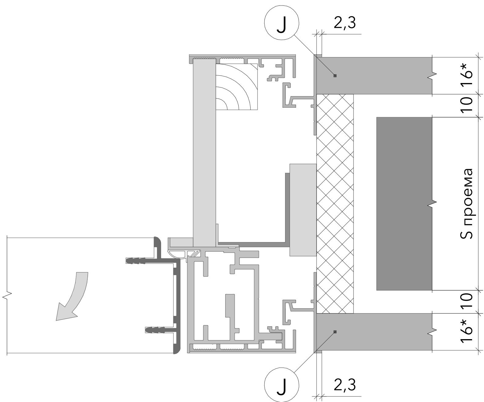
J Теневая коробка Complanar Открытие наружу Конфигурация проема. Тип 1
