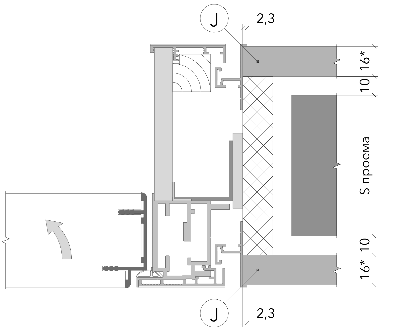
J Теневая коробка Complanar Открытие внутрь Конфигурация проема. Тип 1
