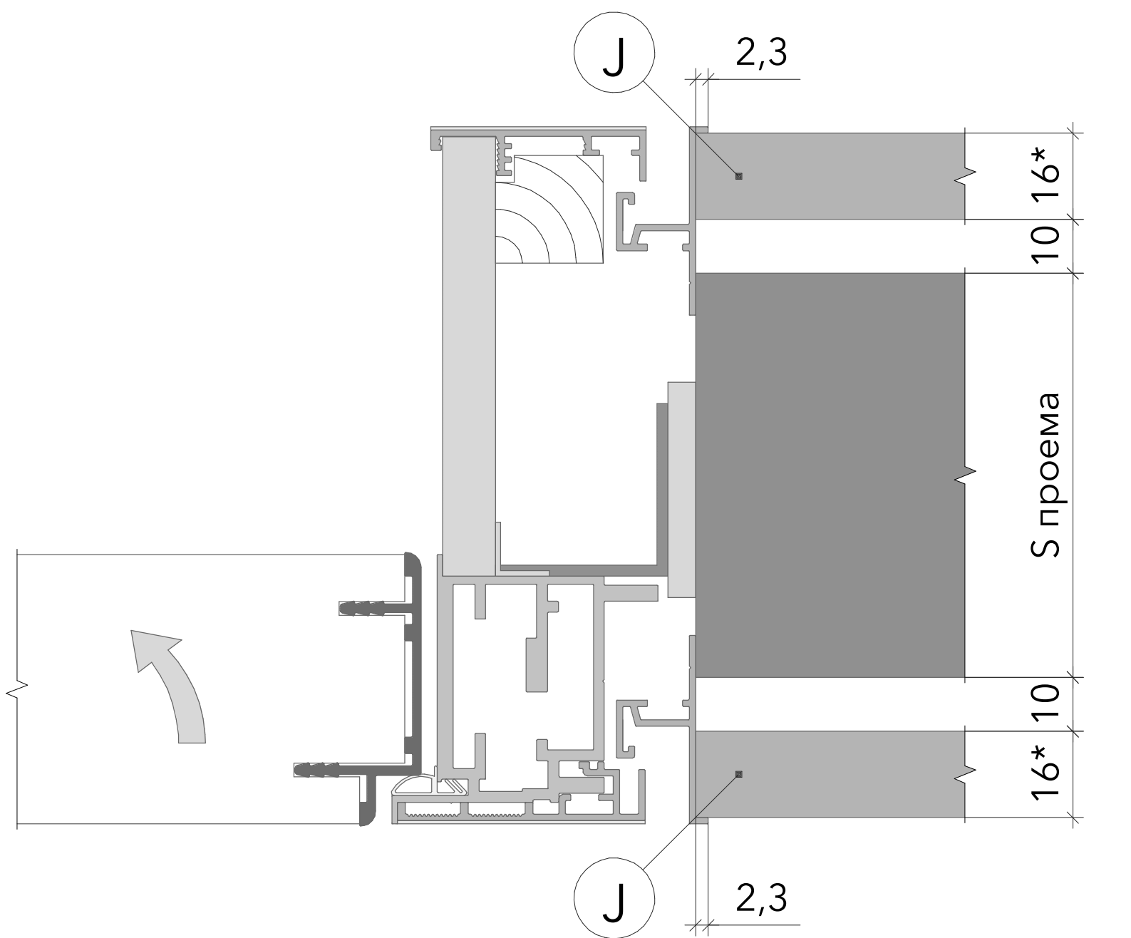
J Теневая коробка Complanar Открытие внутрь Конфигурация проема. Тип 2
