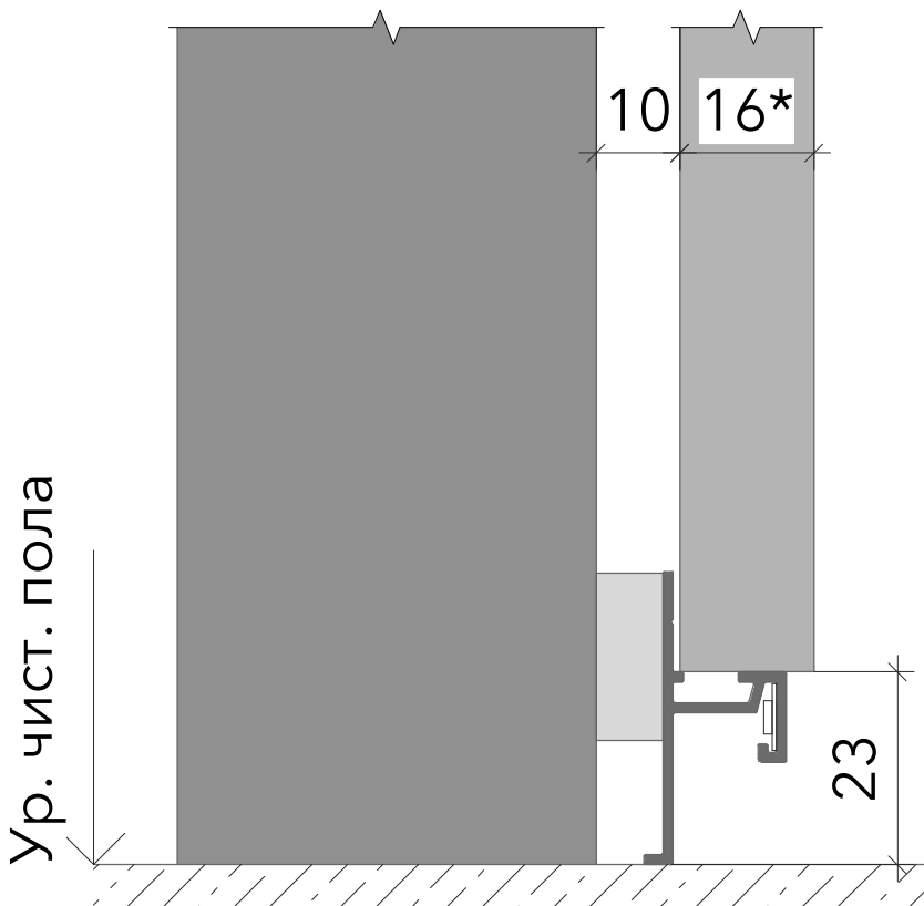
K Теневой плинтус
