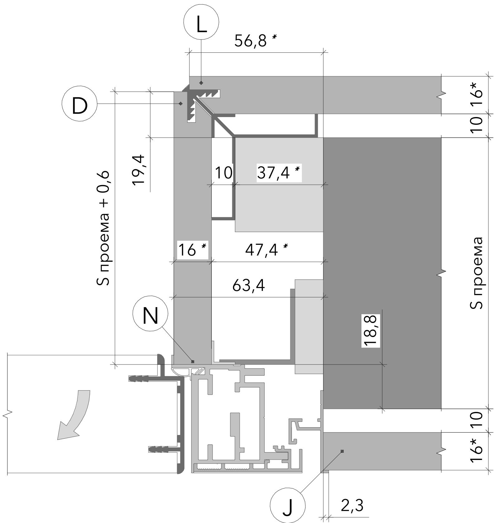
Коробка Complanar 50 Наличник Shade Открытие наружу
