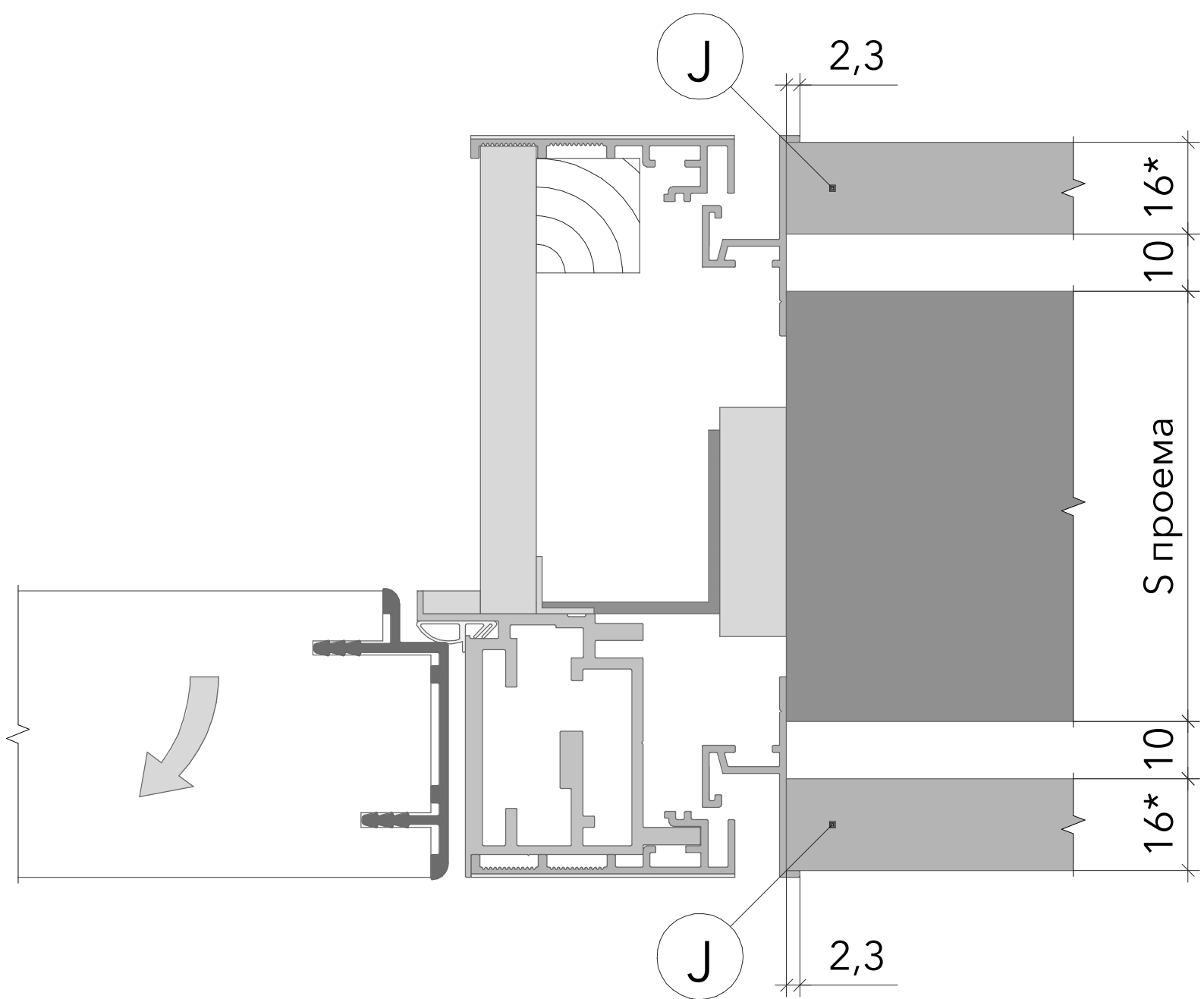
J Теневая коробка Complanar Открытие наружу Конфигурация проема. Тип 2
