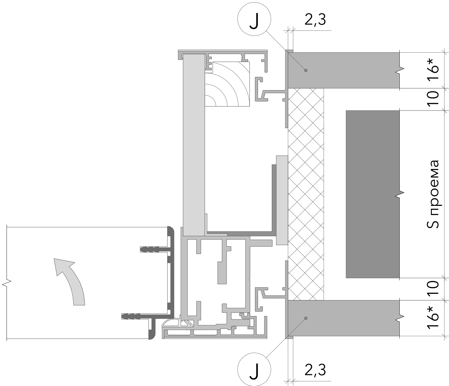
J Теневая коробка Complanar Открытие внутрь Конфигурация проема. Тип 1
