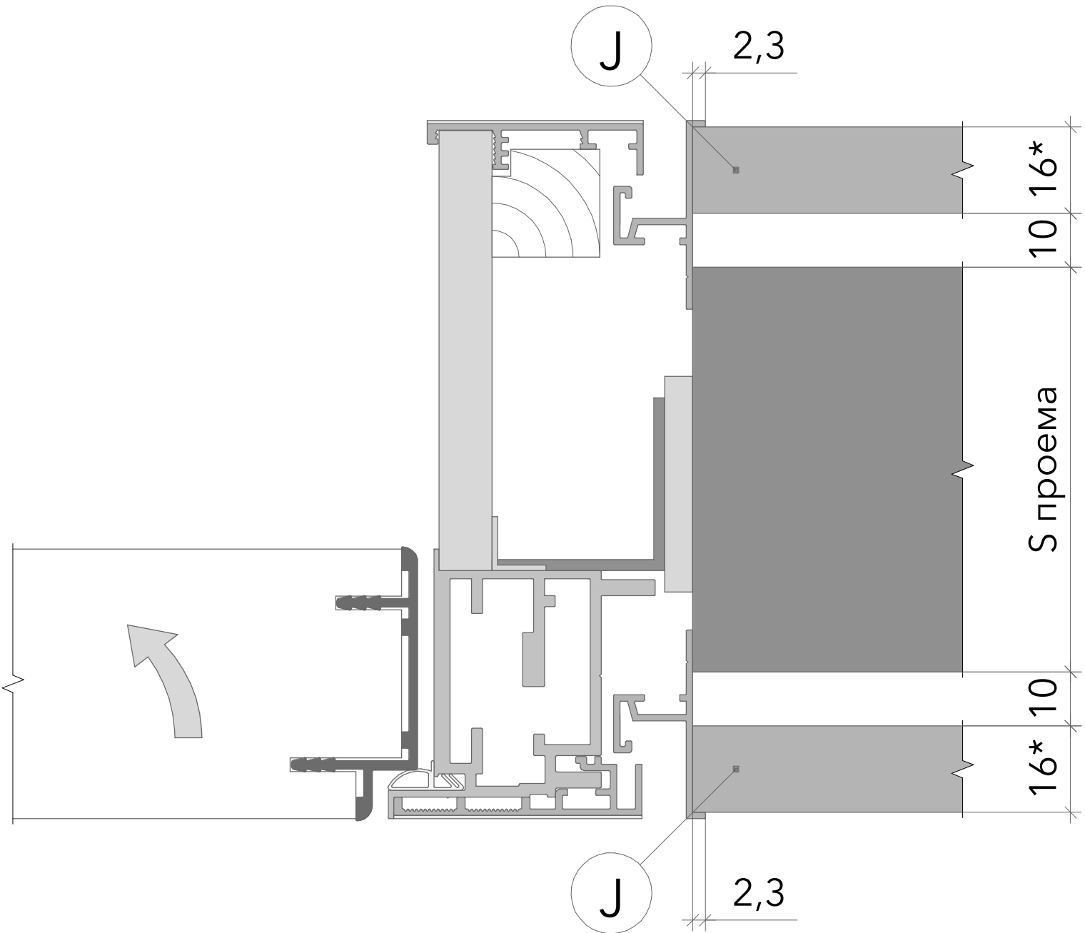
J Теневая коробка Complanar Открытие внутрь Конфигурация проема. Тип 2
