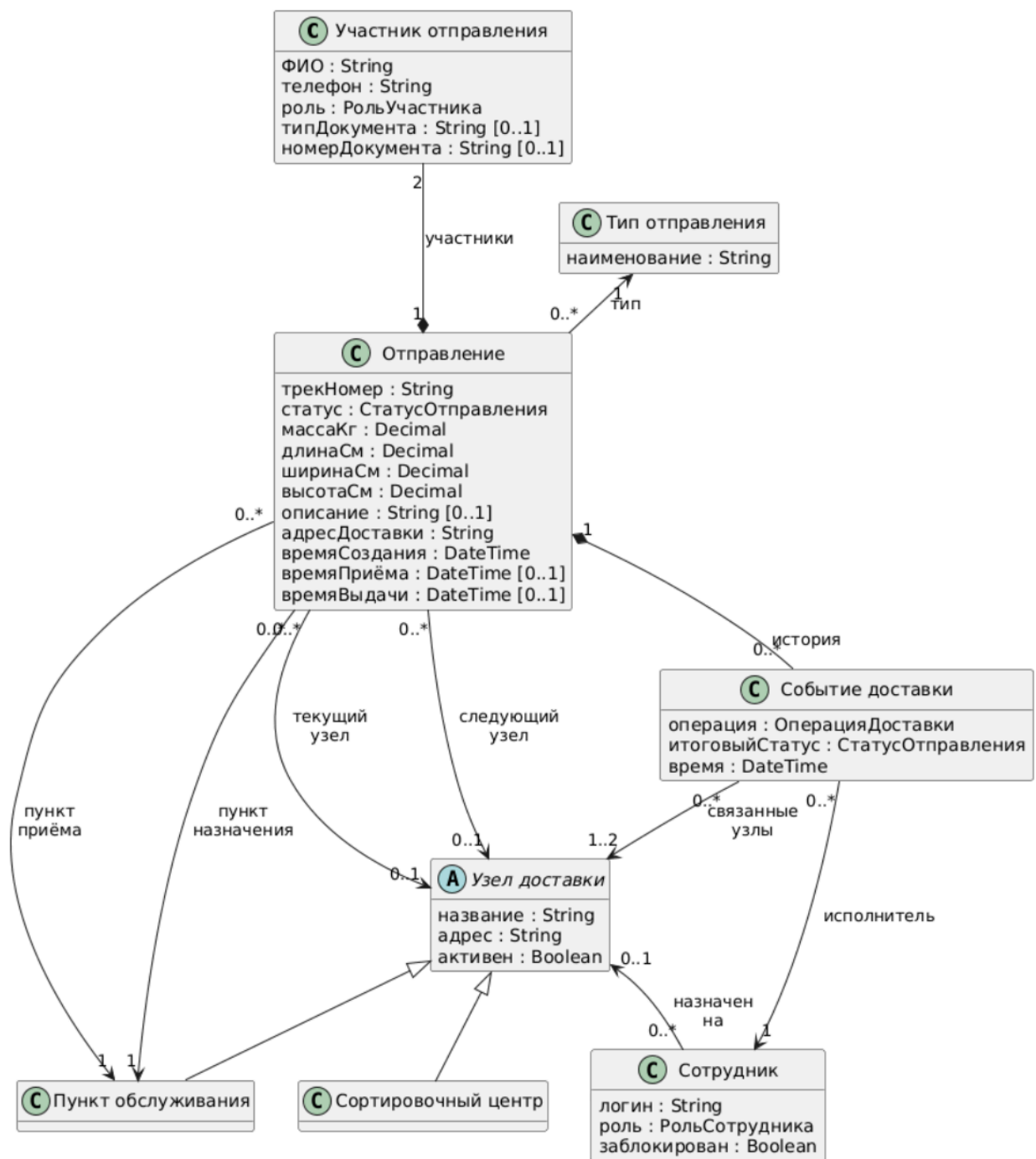
Рис. 4. Диаграмма классов
