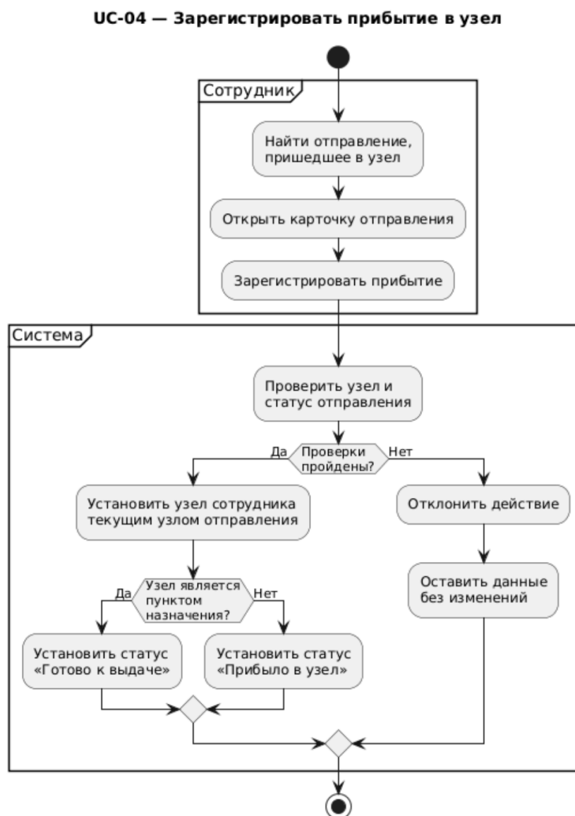
Рис. 2. Диаграмма activity
