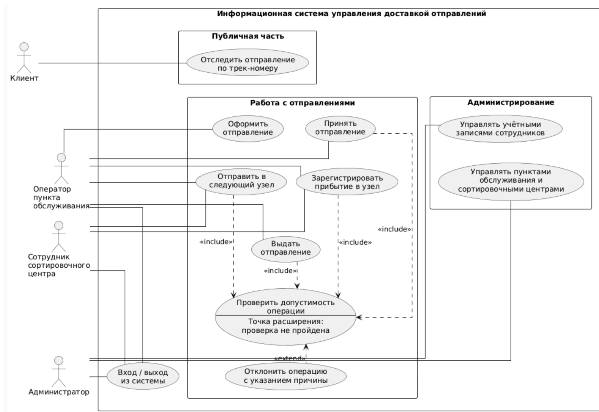
Рис. 3. Диаграмма Use Case уточненная
