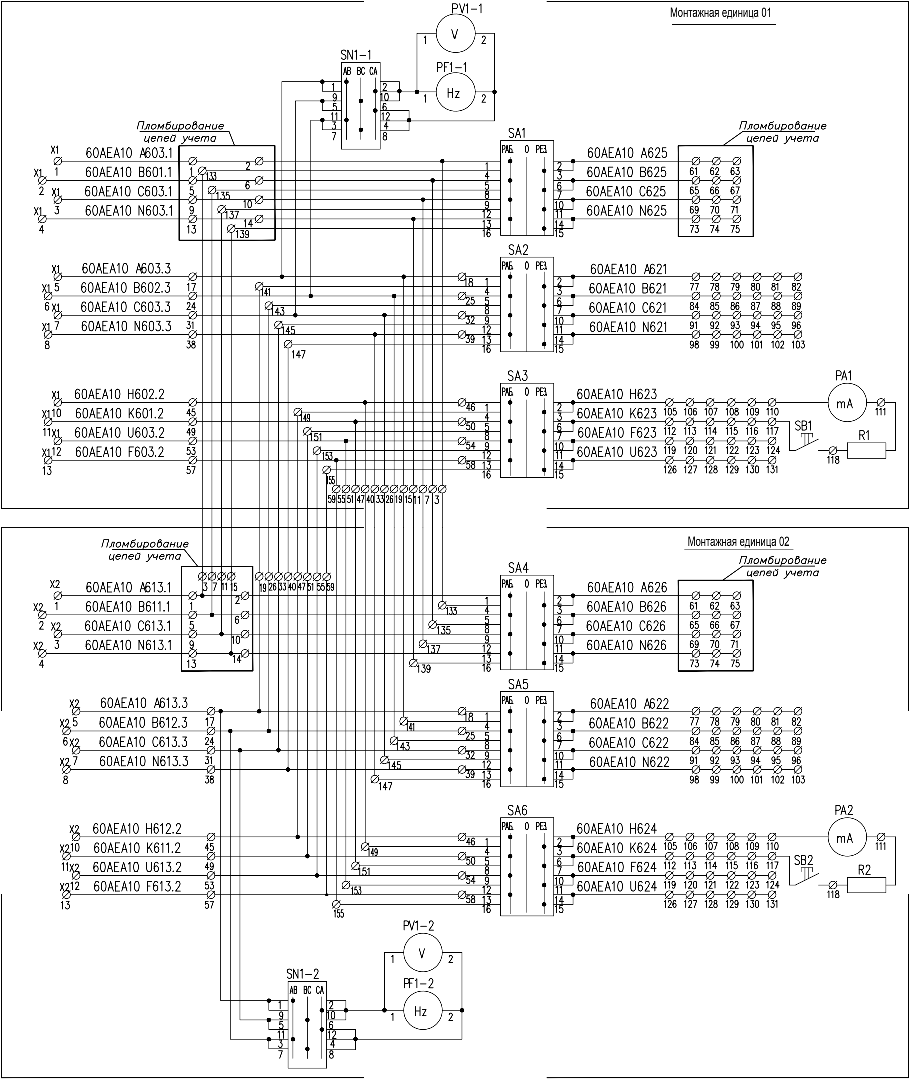
Схема электрическая полная
