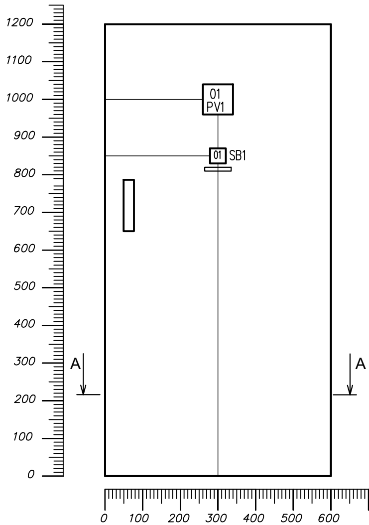
Вид спереди с дверью
