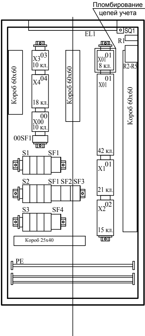
Вид спереди со снятой дверью
