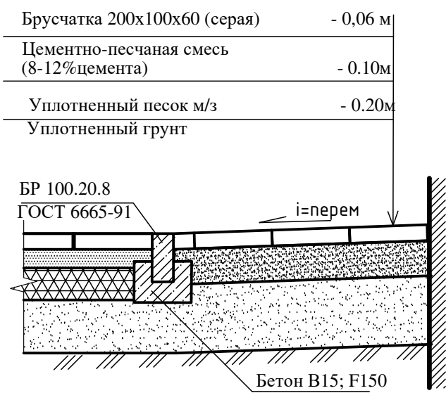
тип 2 Покрытие откоски
