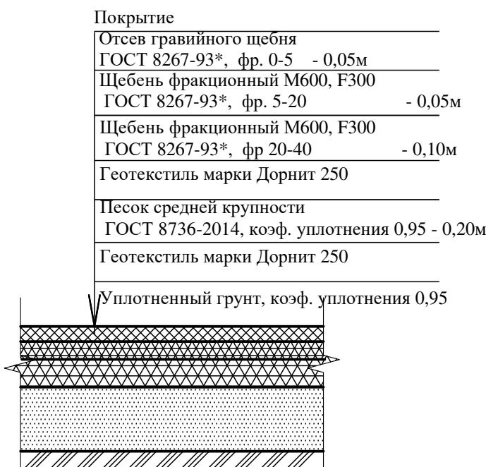
тип 4 Покрытие футбольного поля
