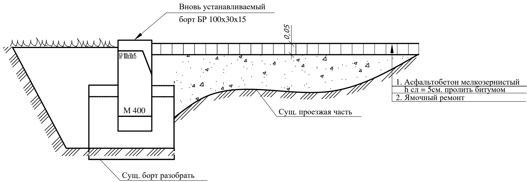
тип 1 Ремонт а/б покрытия проезжей части
