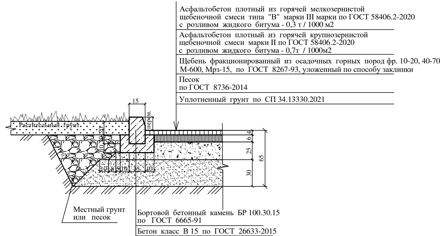
тип 6 Покрытие проезжей части
