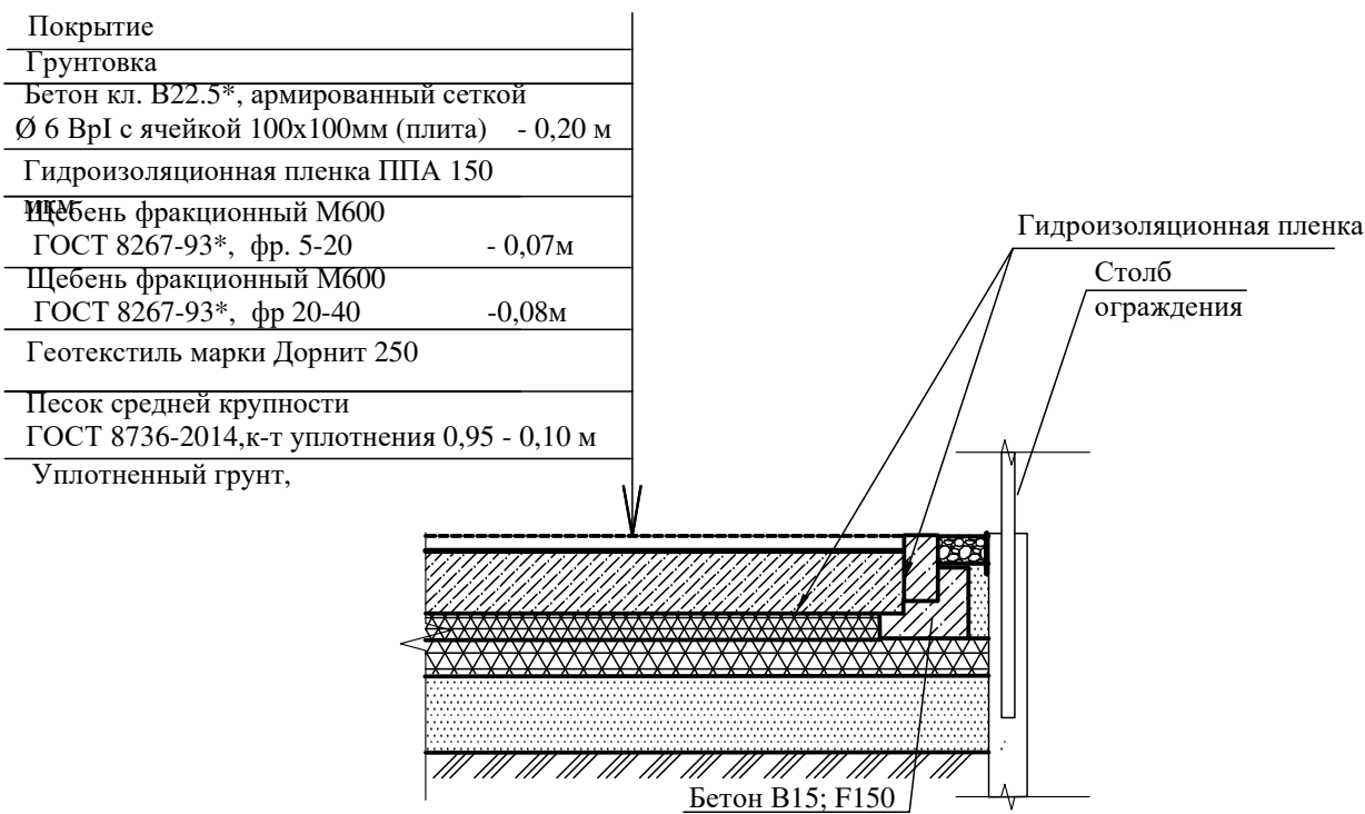
тип 5 Покрытие игровой площадки баскетбол
