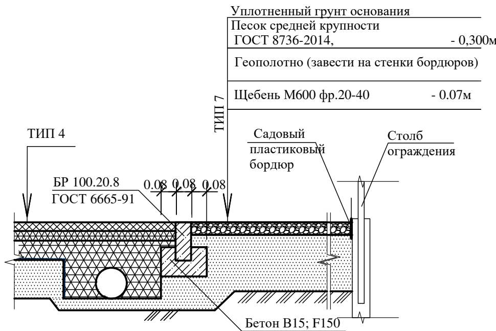
тип 7 Покрытие буферной зоны вокруг футбольного поля
