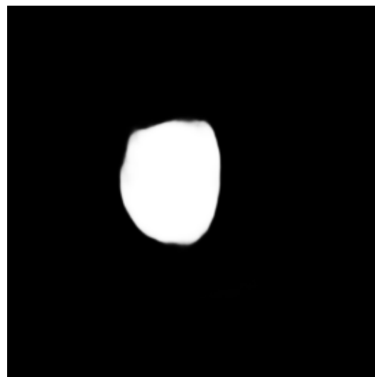
U-Net (RGB)
