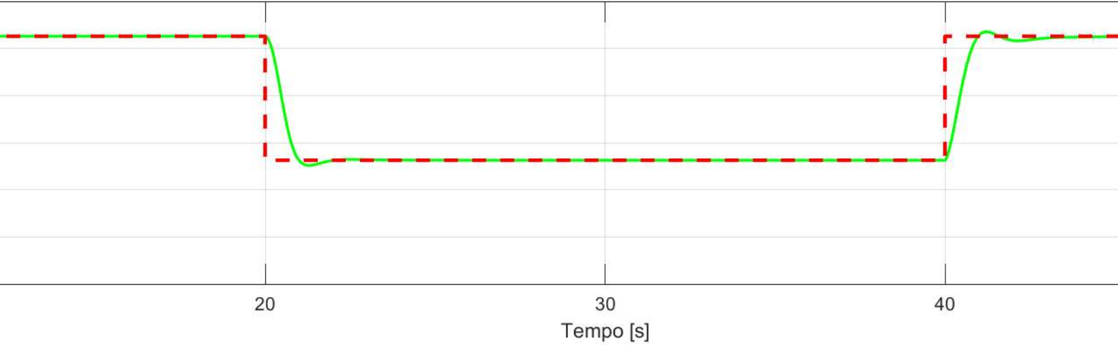
Ensaio resposta ao degrau com U = U_{\text{nominal}} e referência variável
