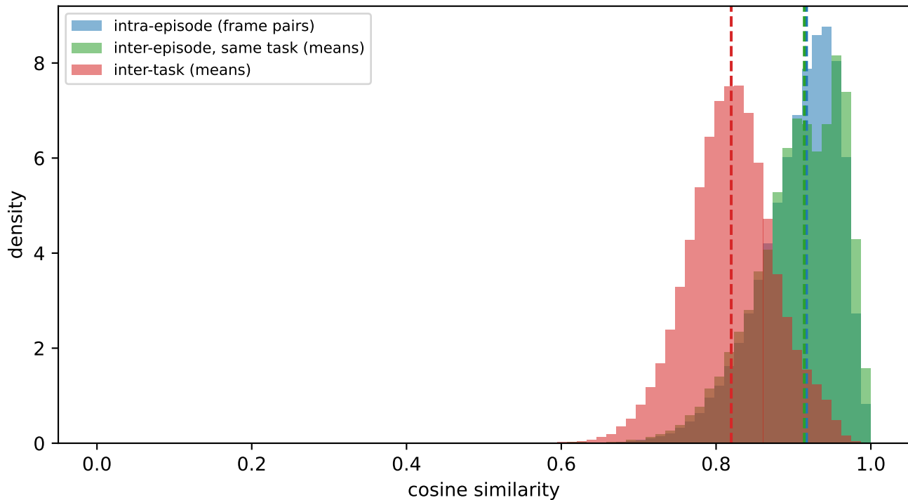
CLIP embedding similarity (20-task)
