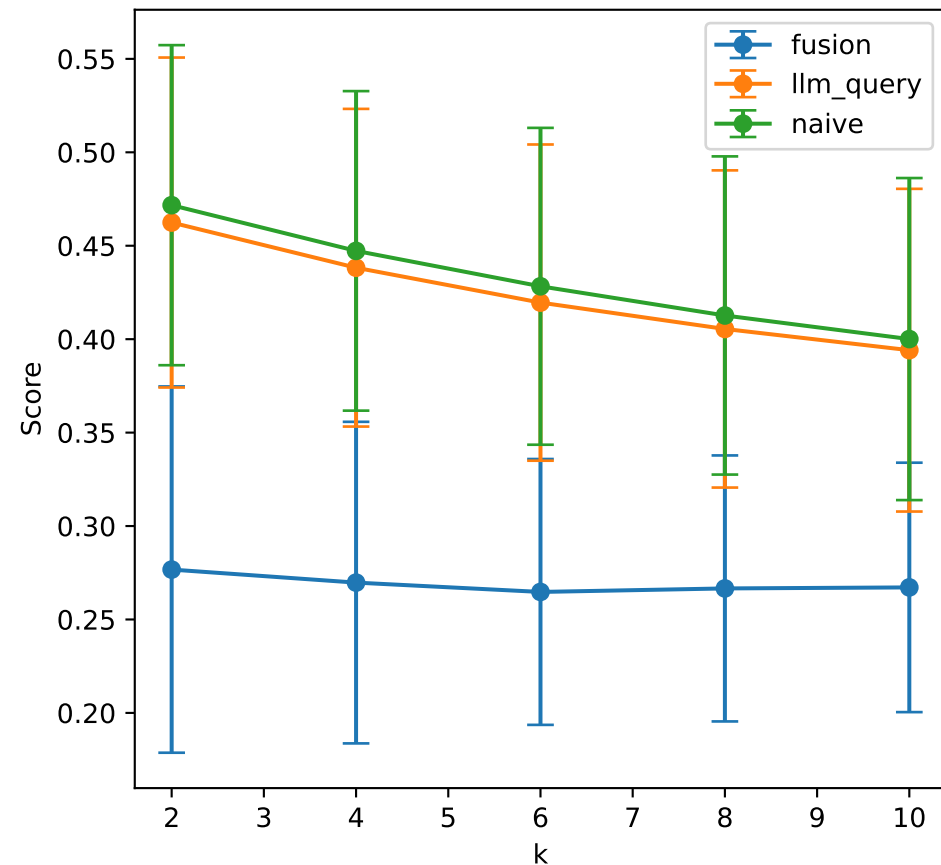
Context Precision
