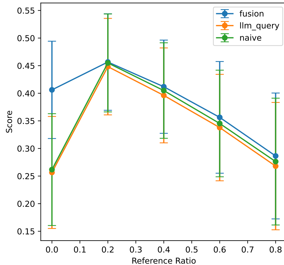
Context Precision
