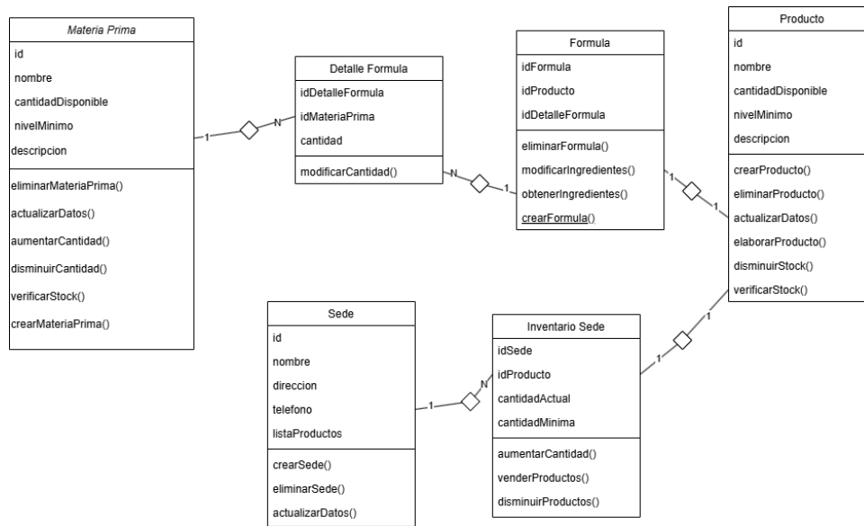
Figura 1: Diagrama de clases del sistema
