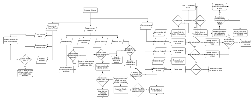
Figura 2: Diagrama de flujo del proceso de producción
