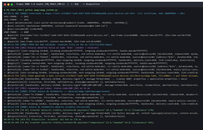
Fig. 6 — Tramas AMQP reales (PN_TRACE_FRM): SASL, open, begin, attach $cbs, flow (crédito 50), transfer put-token → disposition accepted y attach del enlace de telemetría (sesión completa: evidencias/02b).
