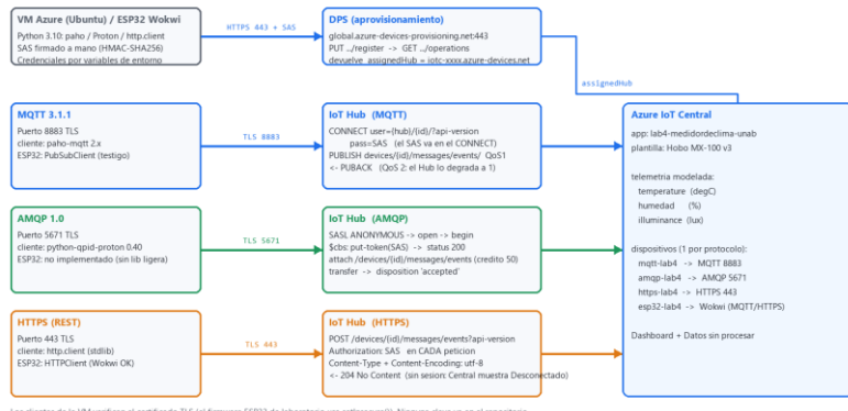
Fig. 1 — Tres caminos hacia IoT Central; DPS por HTTPS en todos.
