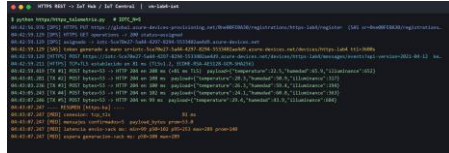
Fig. 7 — Log del cliente HTTPS en la VM: DPS por REST, POST y HTTP 204 por cada lectura (curl: evidencias/11).
