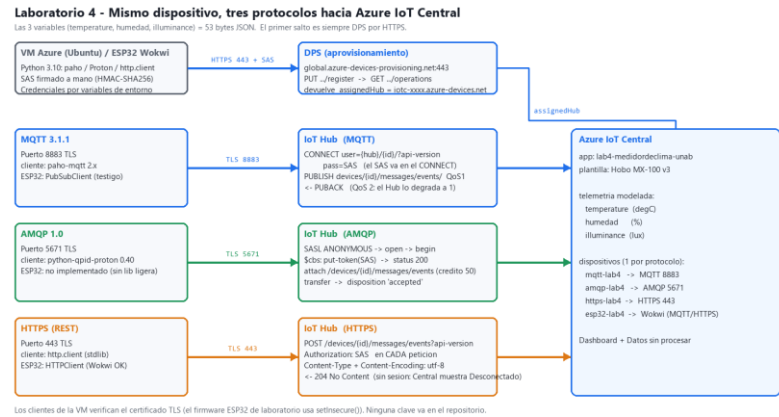
Fig. 1 — Tres caminos hacia IoT Central; DPS por HTTPS en todos.
