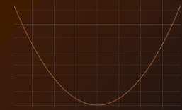
Quadratic
