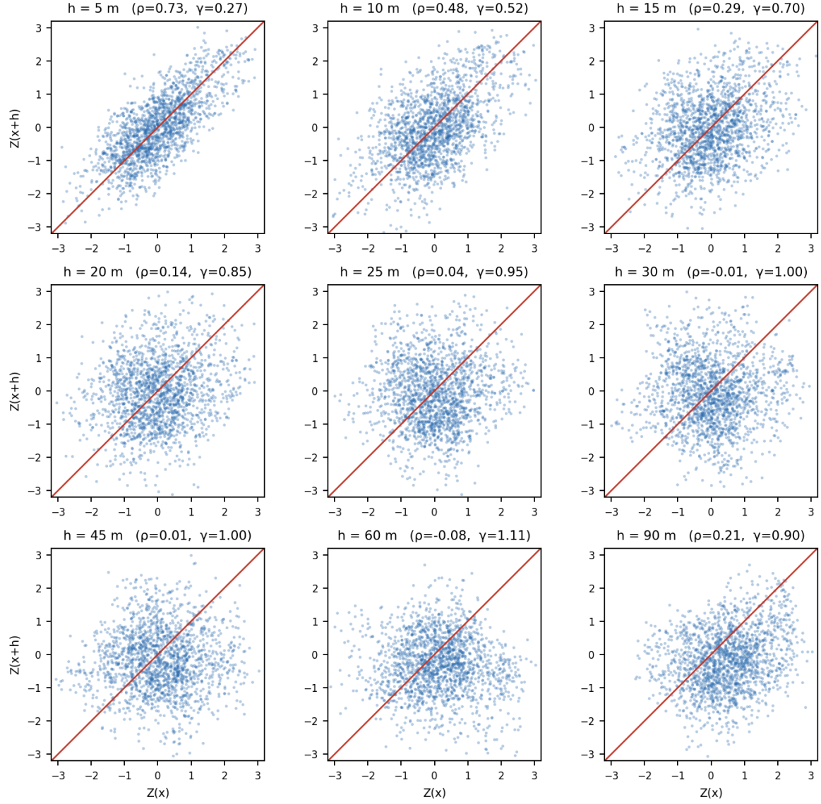
FIGURE 3 : Nuage de Z(\mathbf{x}) en fonction de Z(\mathbf{x}+\mathbf{h}) pour des distances croissantes, calculé sur un champ gaussien isotrope de modèle sphérique et de portée 30 m. Lorsque la distance augmente, le nuage s'éloigne progressivement de la diagonale, la corrélation diminue et le variogramme augmente.
