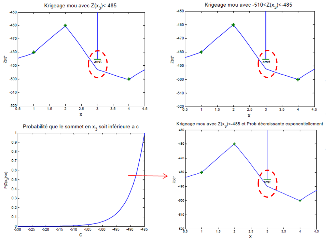
FIGURE 7 : Résultats du krigage d'indicateurs avec une donnée d'inégalité et des données souples.
