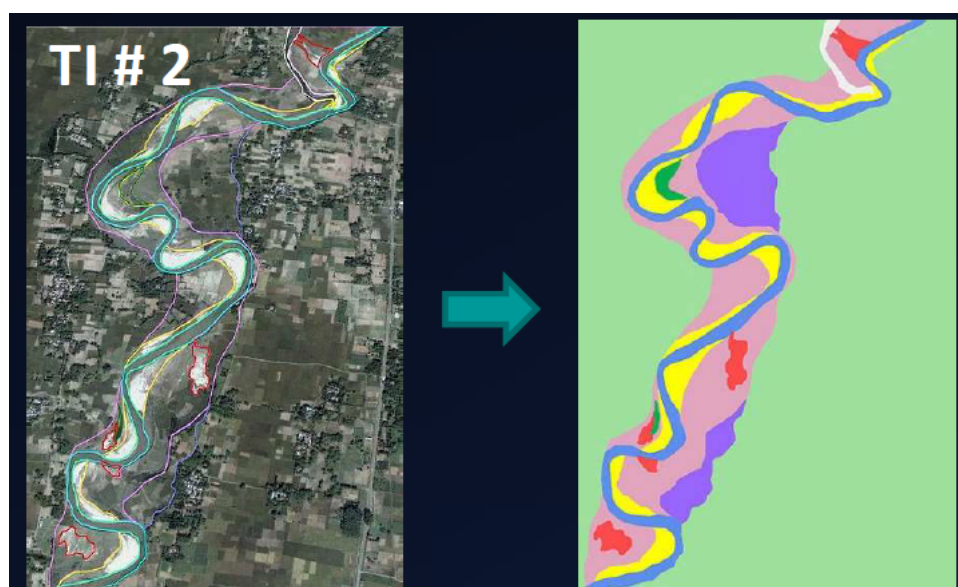
FIGURE 19 : Image d'entraînement n° 2 — chenal méandrique extrait d'une image satellite : la réalisation restitue la sinuosité et les recouvrements de méandres.
