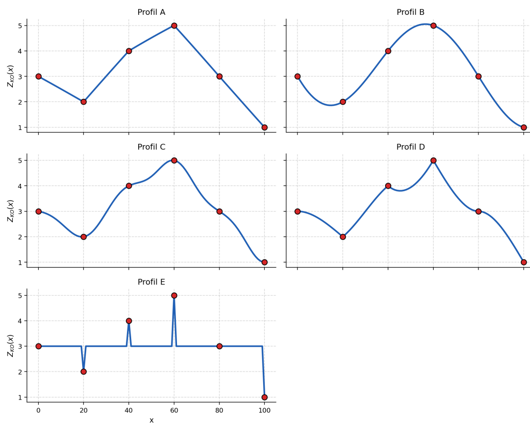
FIGURE 6 : Profils de krigage à associer à leur modèle de covariance : la forme du profil (lissage, portée, pépité) trahit le modèle.
