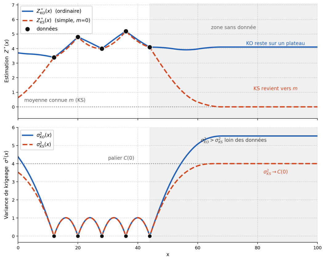
FIGURE 2 : Profils de krigeage simple (KS) et ordinaire (KO) : loin des données, le KS revient vers la moyenne connue tandis que le KO reste sur un plateau ; la variance du KS plafonne au palier.
