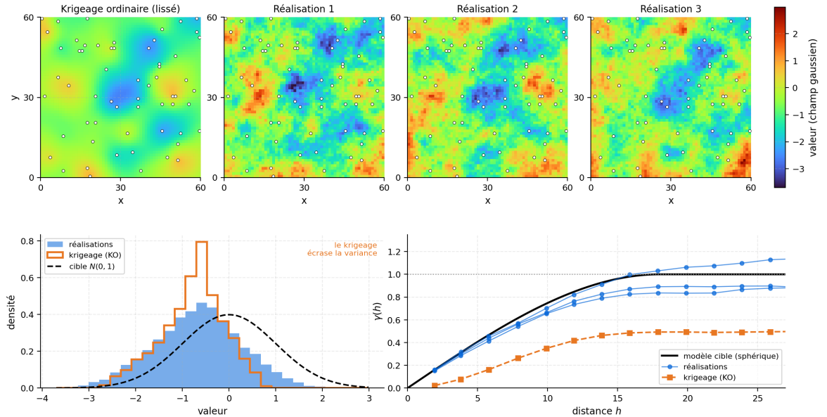
FIGURE 2 : Krigeage lissé vs réalisations conditionnelles : les réalisations reproduisent l'histogramme et le variogramme du modèle, contrairement au krigeage qui écrase la variance.
