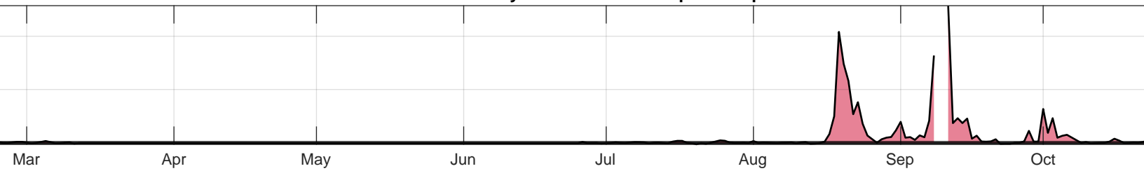
BEUTI
