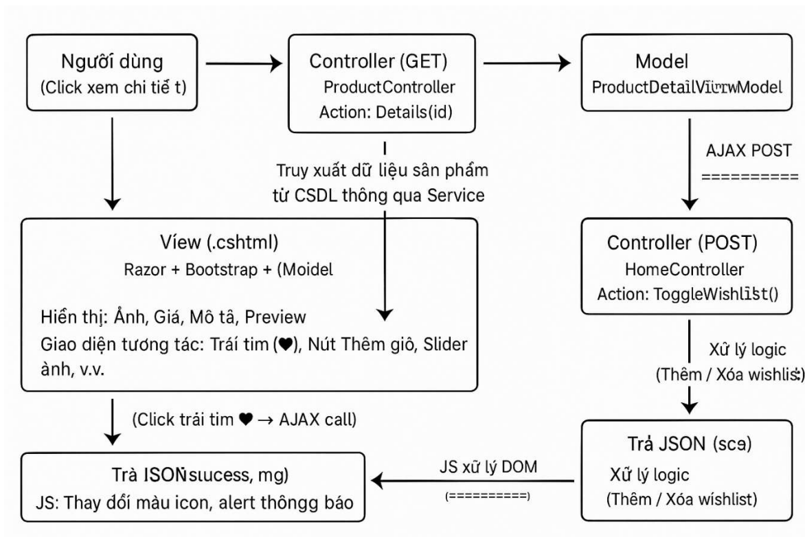
Hình 2.13: Sơ đồ minh họa cấu trúc hoạt động của dự án
