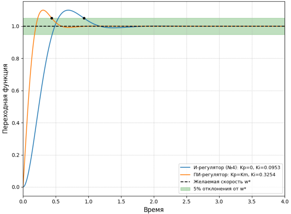
Рис. 16: Сравнение наилучшего И-регулятора (п. 2.3) и оптимального ПИ-регулятора
