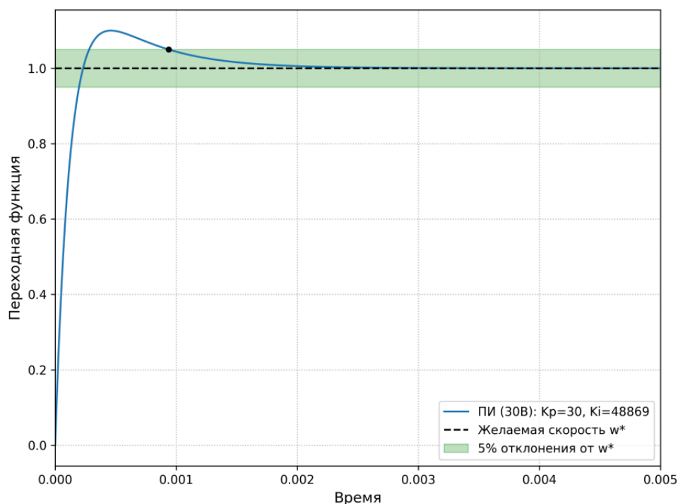
Рис. 17: ПИ-регулятор с ограничением управляющего напряжения 30В
