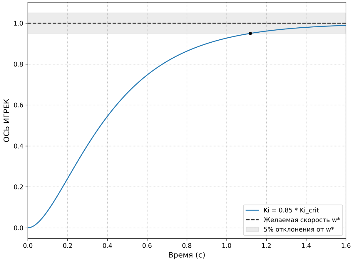
Рис. 9: График переходной функции при разных вещественных корнях
