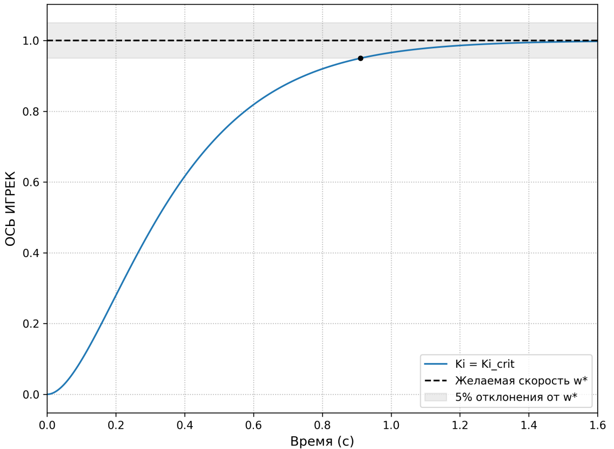
Рис. 10: График переходной функции при кратном вещественном корне
