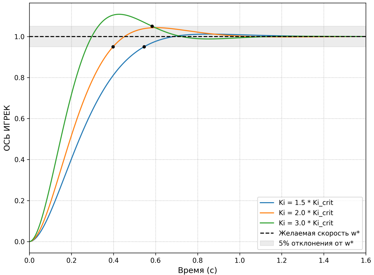
Рис. 11: График переходной функции при комплексных корнях
