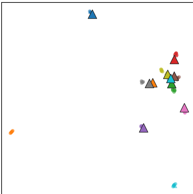
MIL-CREDA*
