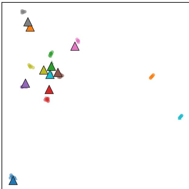
MIL-Baseline
