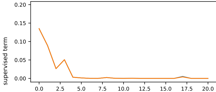
U-&gt;M
