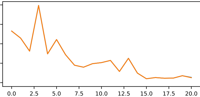
S-&gt;M
