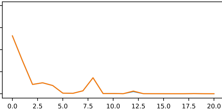
M-&gt;U
