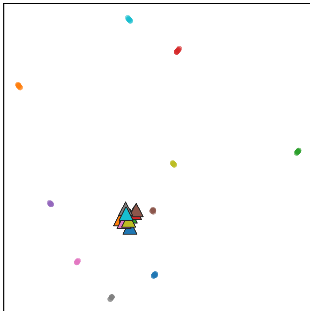
MIL-Baseline
