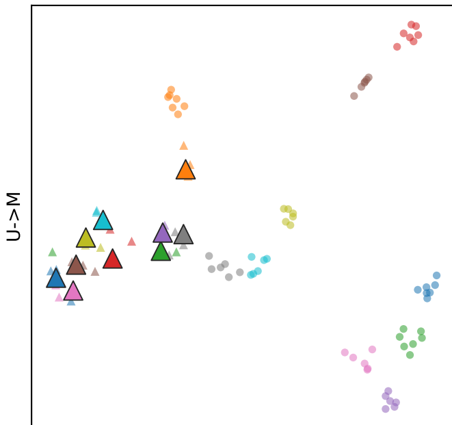
MIL-Baseline
