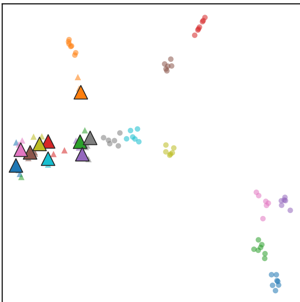
MIL-CREDA*
