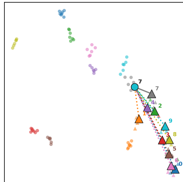
MIL-CREDA
