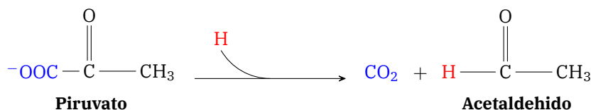
Figura 2.4: Reacción catalizada por la piruvato descarboxilasa (EC 4.1.1.1). Esta retira el grupo carboxilo ( \text{COOH} ), reacción llamada descarboxilación y de donde proviene el nombre descarboxilasa. Tras esto un átomo de hidrógeno toma el lugar del grupo carboxilo.
