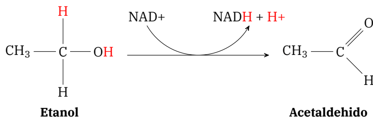
Figura 2.1: Reacción catalizada por la alcohol deshidrogenasa (EC 1.1.1.). Aquí la enzima utiliza el \text{NAD}^+ como cofactor para oxidar el etanol, esto al eliminar de este 2 átomos de hidrógeno y 2 electrones, lo que transforma al etanol en acetaldehído. La alcohol deshidrogenasa está presente en nuestro hígado, y hoy día el principal uso que hacemos de ella es para el metabolismo de bebidas alcohólicas.
