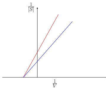
(c) Inhibición no competitiva
