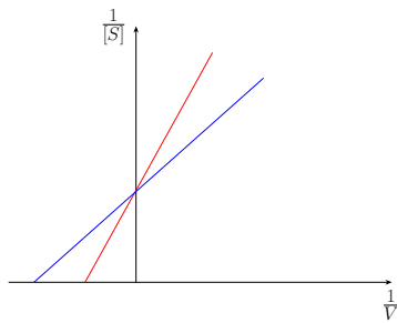
(a) Inhibición competitiva
