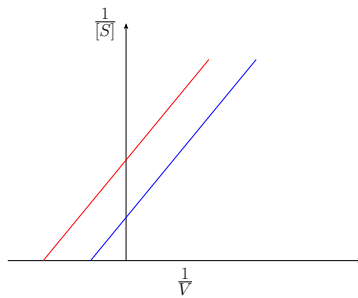
(b) Inhibición incompetitiva
