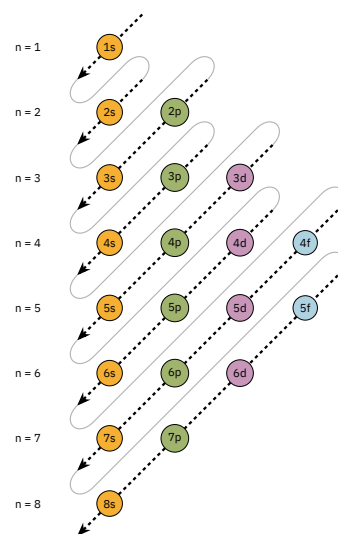
Figura 2.1: Esquema de niveles de energía
