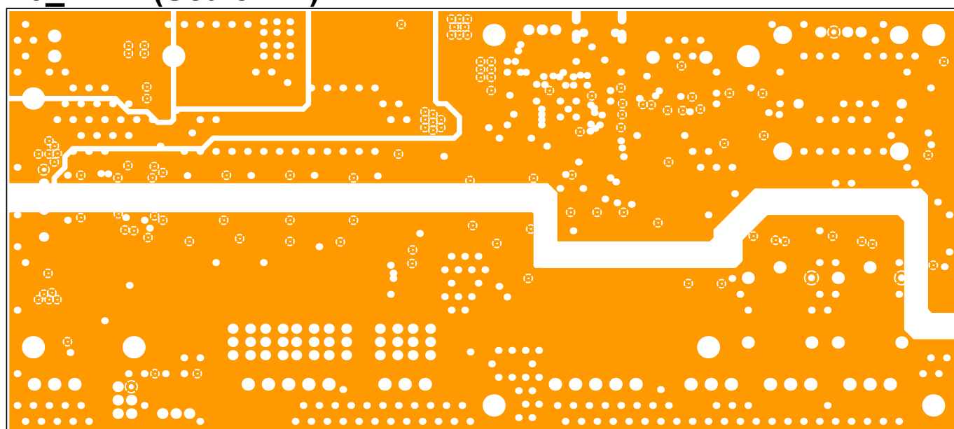
L3_PWR (Scale 1:1)
