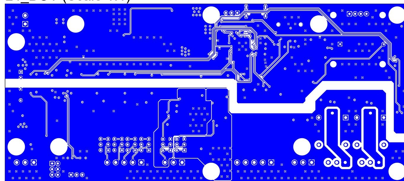
L4_BOT (Scale 1:1)
