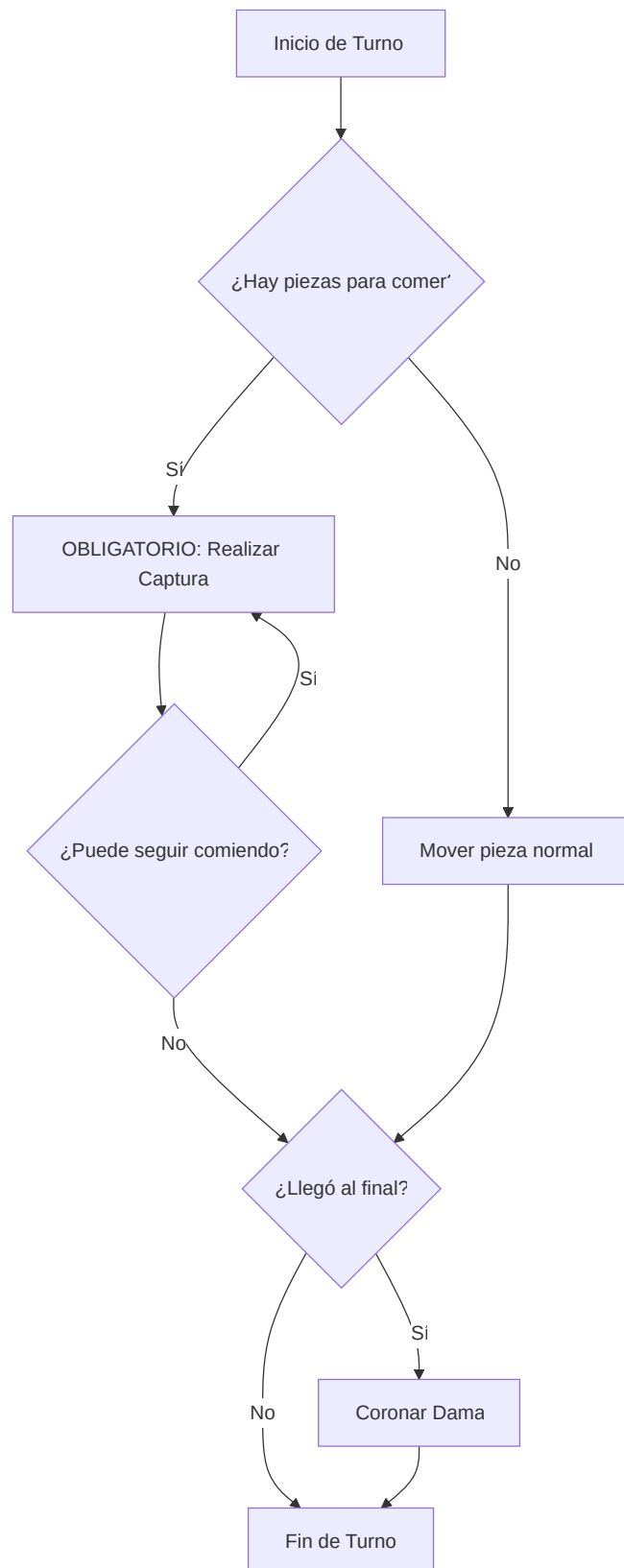
Figura 1. Diagrama de Flujo: Lógica de Turno y Capturas
