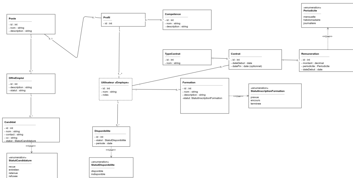
FIGURE 2 – Diagramme de classes métier, Module 3 Profils & RH
