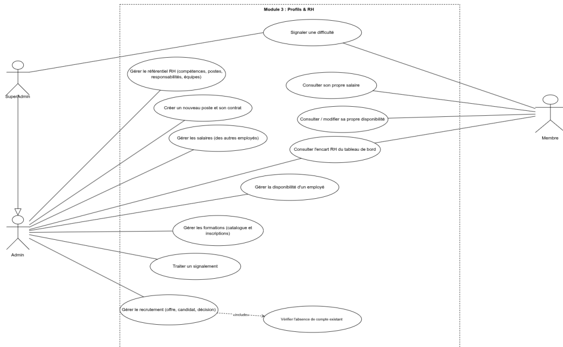
FIGURE 1 – Diagramme de cas d'utilisation, Module 3 Profils &amp; RH
