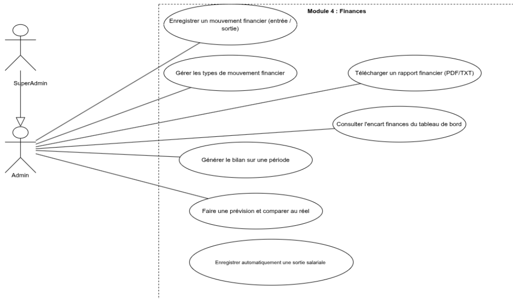
FIGURE 3 – Diagramme de cas d'utilisation, Module 4 Finances
