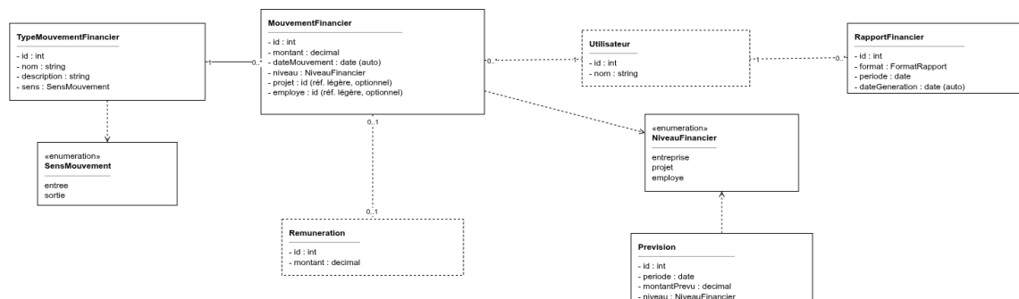
FIGURE 4 – Diagramme de classes métier, Module 4 Finances
