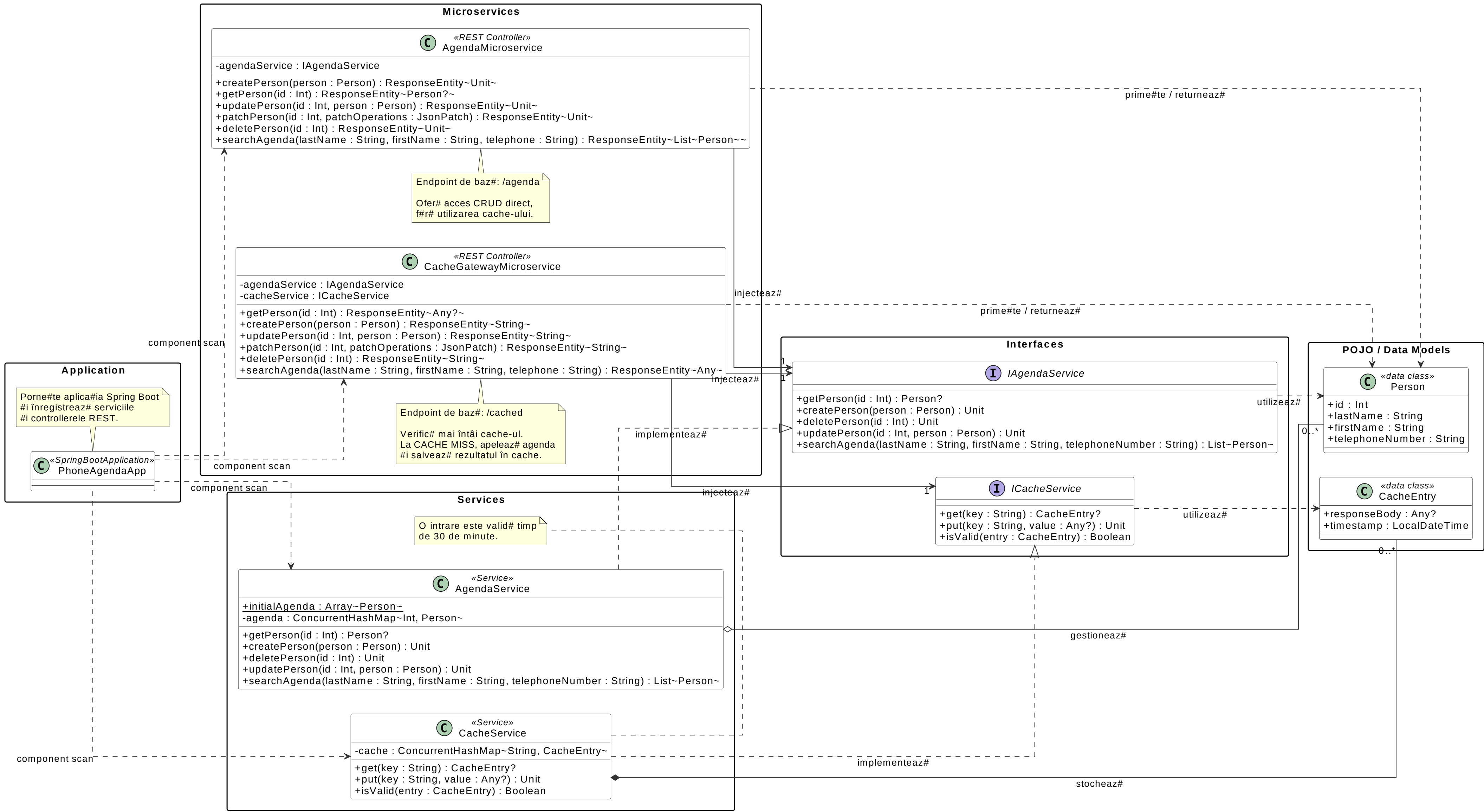
Diagrama de clase - PhoneAgendaWithCache
