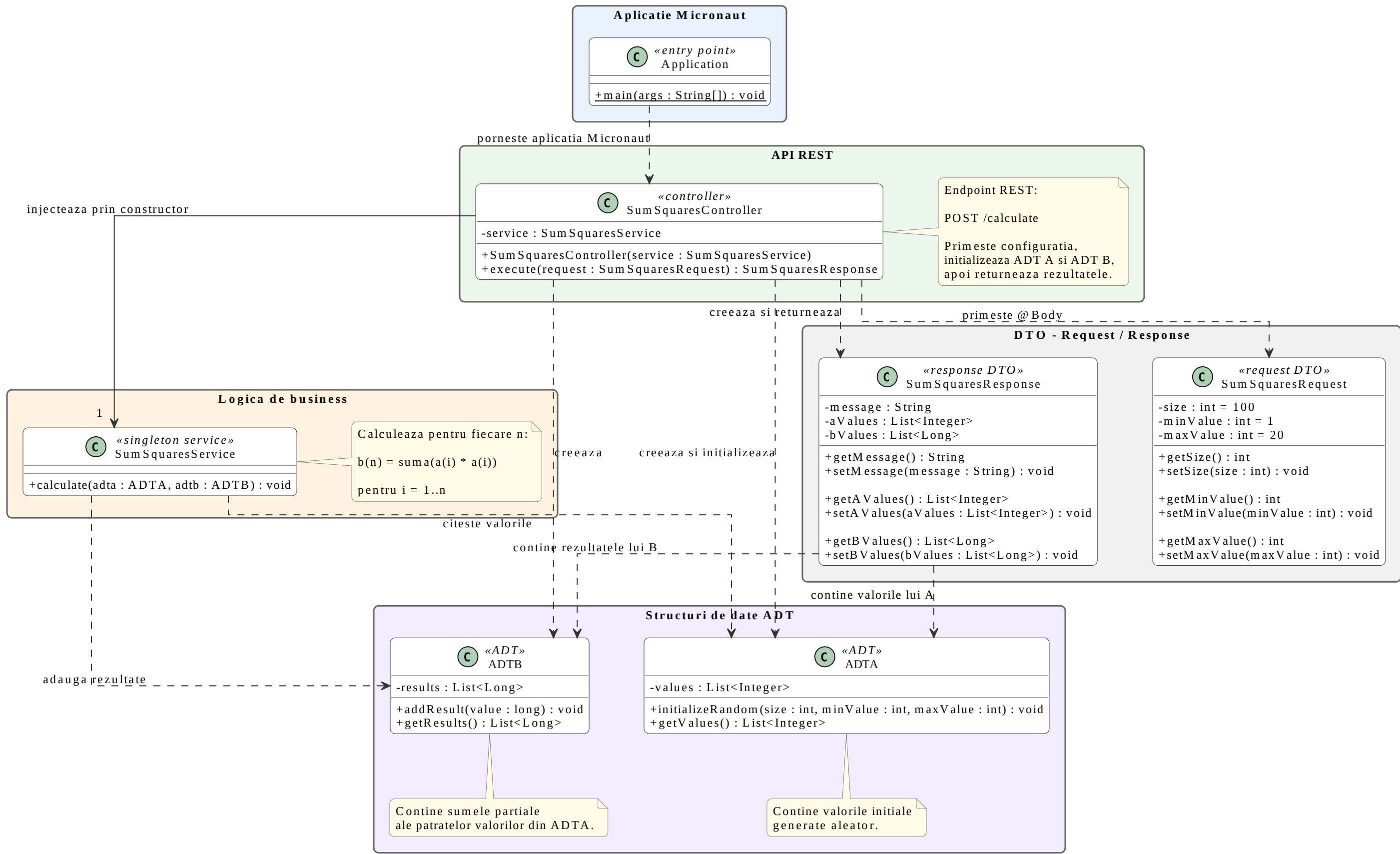
Diagrama de clase - Calculul sumelor parțiale de patrate
