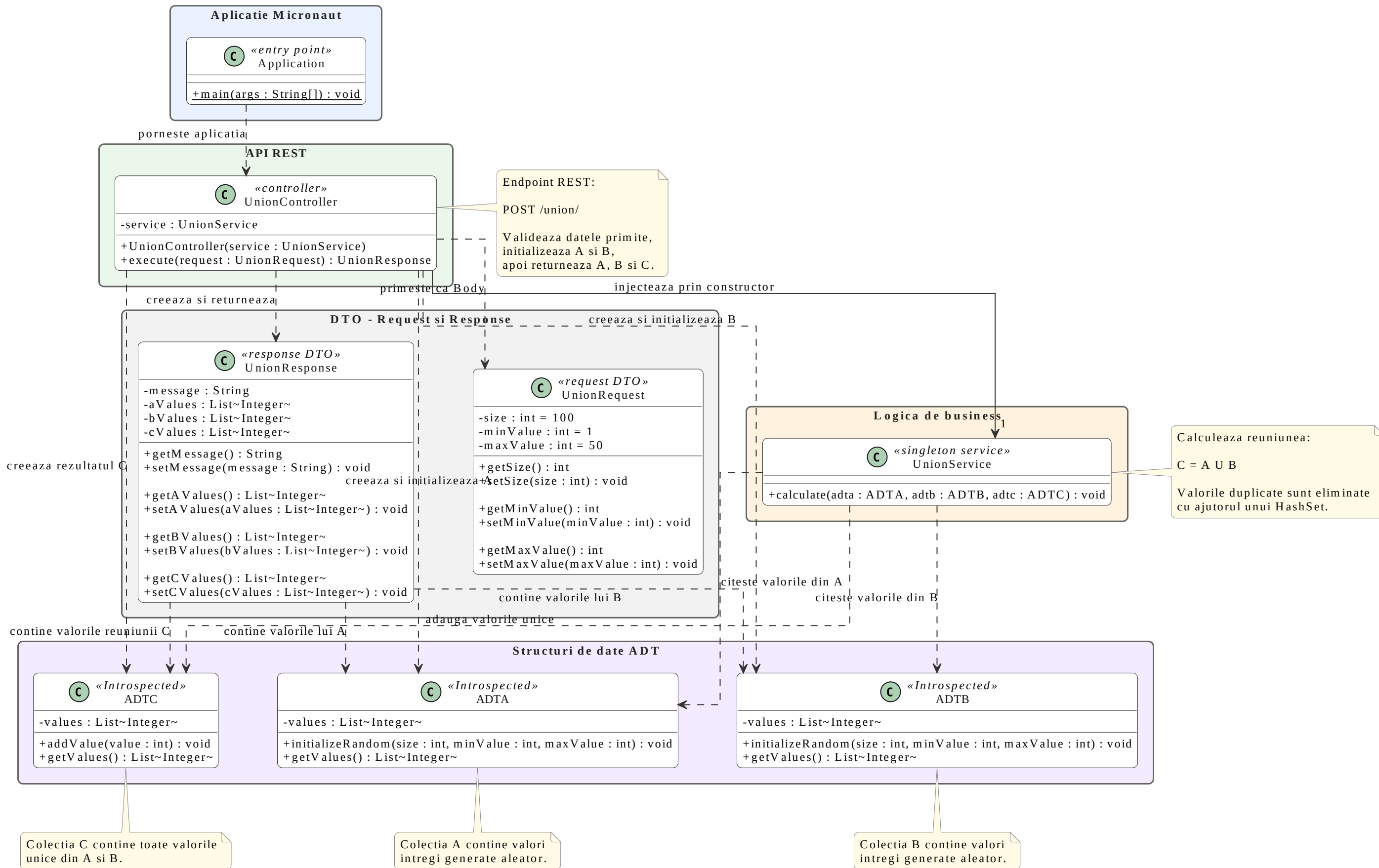
Diagrama de clase - Reuniunea colectiilor A si B
