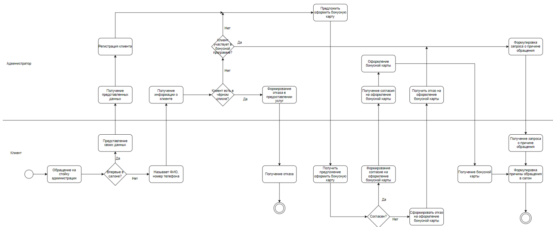
Рис. 6: BPMN
