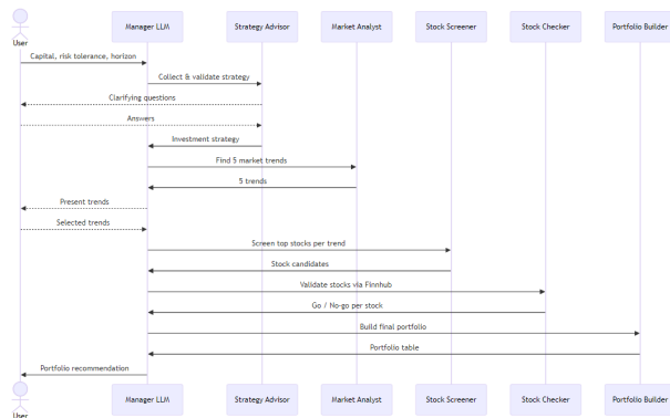
Fig. 2. Interaktionsablauf. Das Manager-LLM delegiert die Tasks sequenziell: Strategieformulierung, Trenderkennung (beide mit menschlichem Input), Aktien-Screening, Validierung über Finnhub und Portfolioerstellung.
