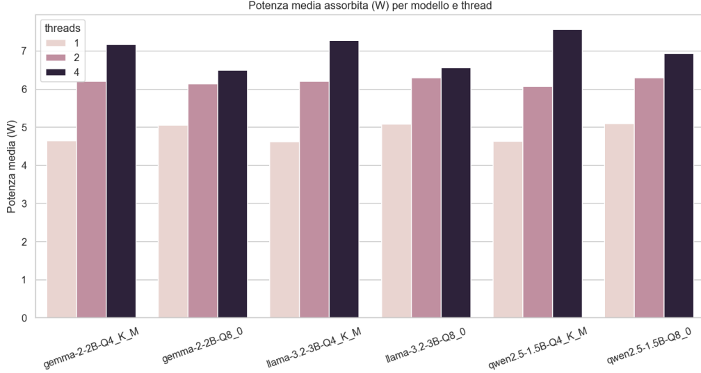
Figura 4.10: Potenza media assorbita al variare del numero di thread (Campagna B).
