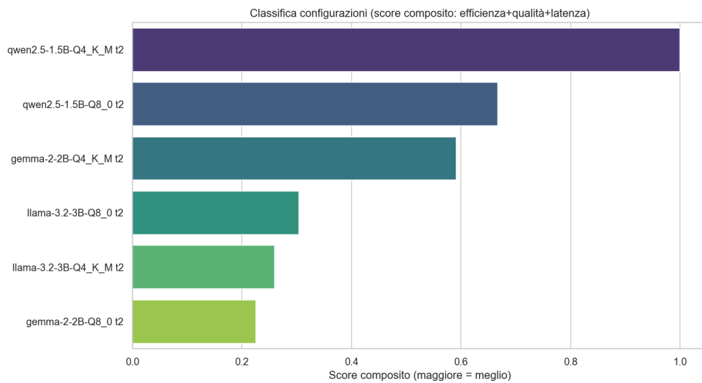
Figura 4.11: Classifica complessiva dei sei modelli secondo lo score composito (Campagna A, a 2 thread).
