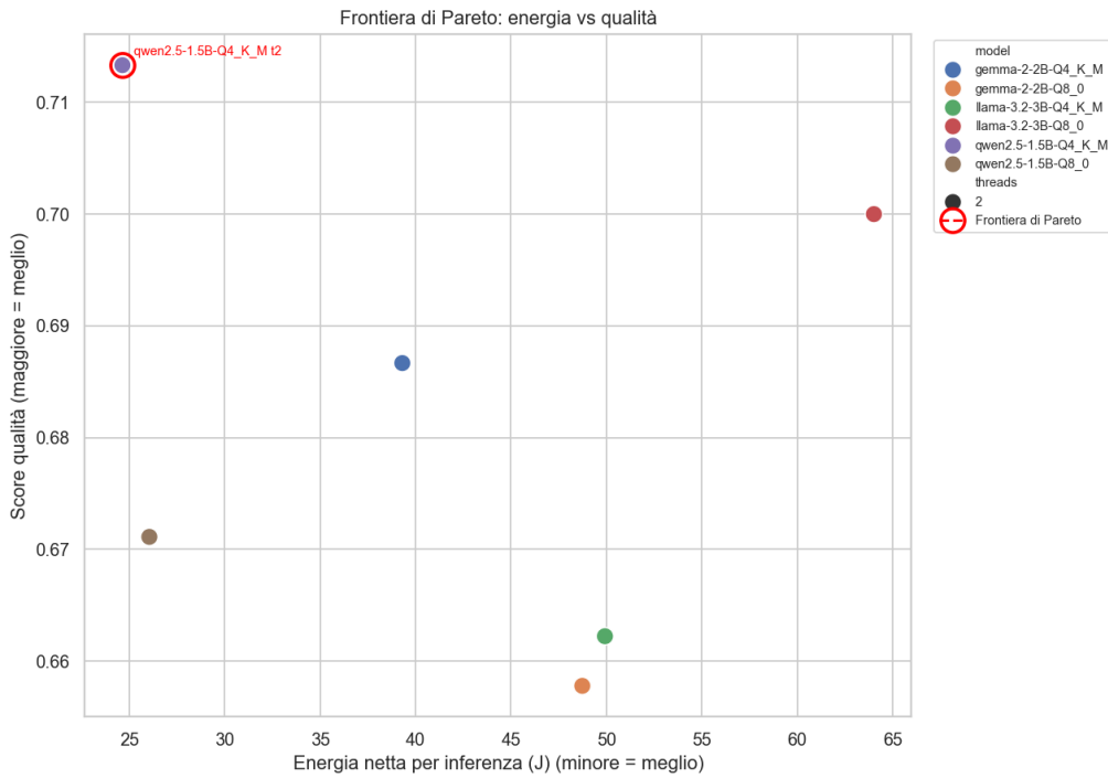
Figura 4.7: Frontiera di Pareto nel piano energia–qualità (Campagna A, i sei modelli a 2 thread; cerchiare in rosso le configurazioni non dominate).
