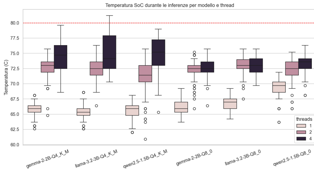
Figura 4.12: Distribuzione della temperatura del SoC durante le inferenze della Campagna B, che comprende le configurazioni a 4 thread, termicamente più impegnative.
