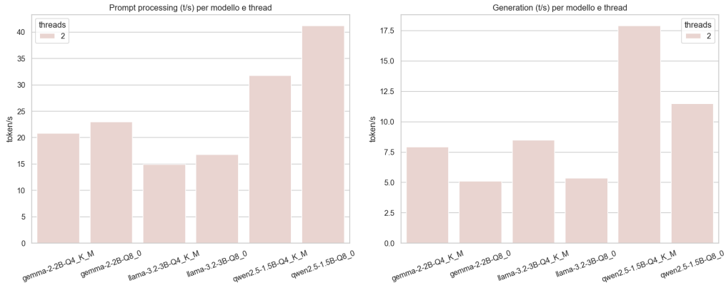
Figura 4.4: Velocità di elaborazione (prompt e generazione) per modello (Campagna A).
