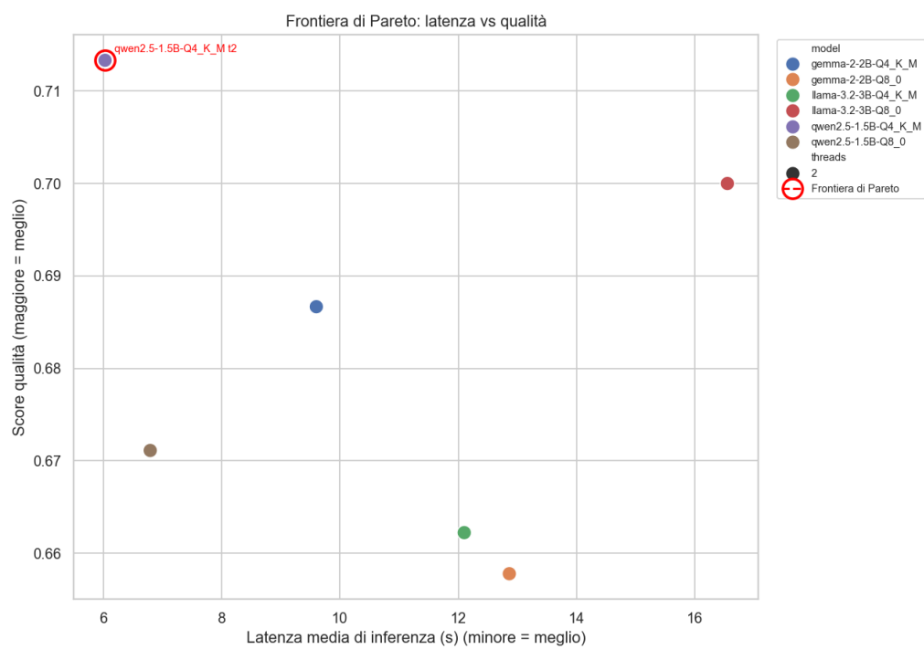
Figura 4.8: Frontiera di Pareto nel piano latenza–qualità (Campagna A, i sei modelli a 2 thread).
