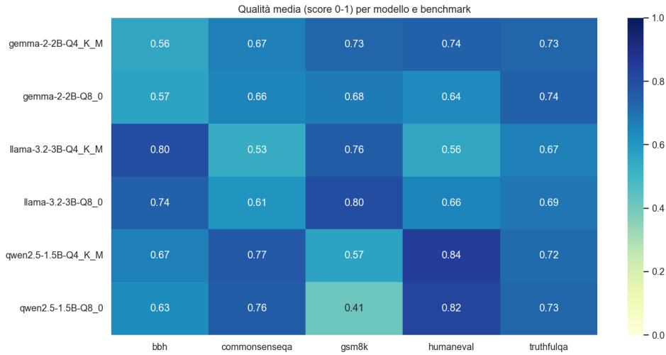
Figura 4.3: Qualità delle risposte (accuratezza media) per modello e benchmark (Campagna A).
