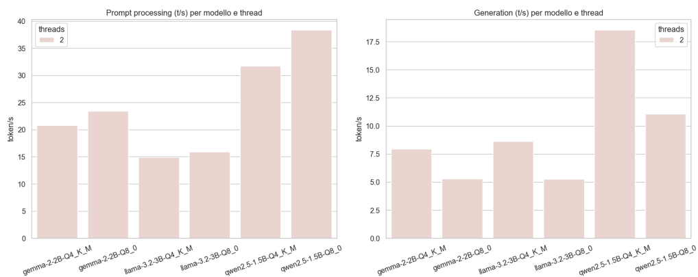
Figura 4.4: Velocità di elaborazione (prompt e generazione) per modello (Campagna A).
