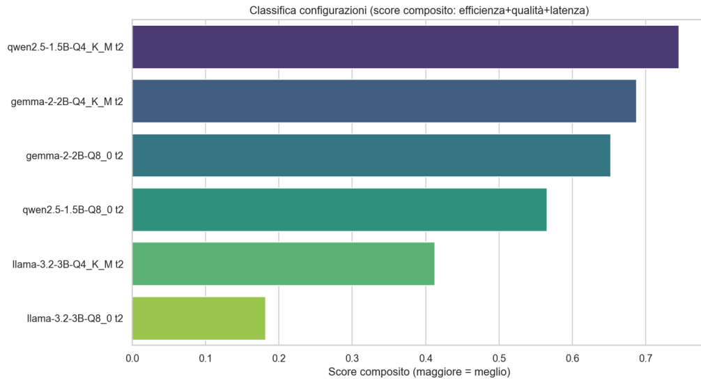
Figura 4.10: Classifica complessiva delle configurazioni secondo lo score composito.
