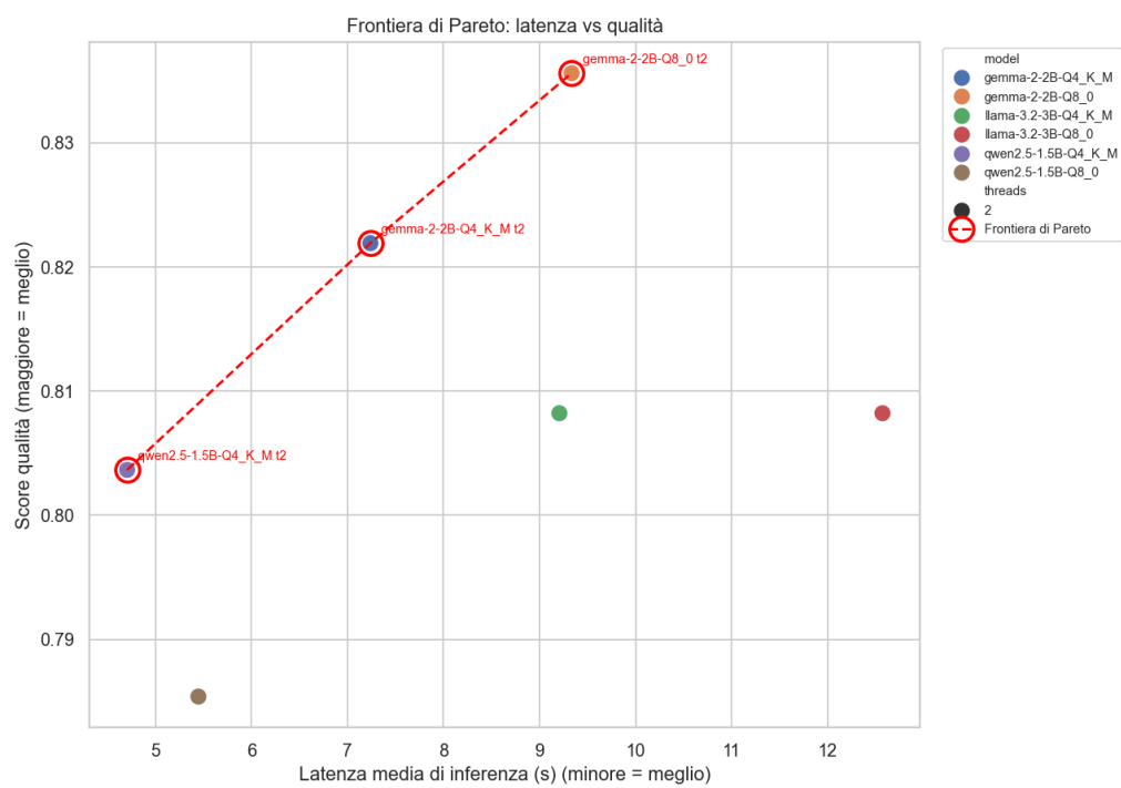
Figura 4.7: Frontiera di Pareto nel piano latenza–qualità (Campagna A, i sei modelli a 2 thread).
