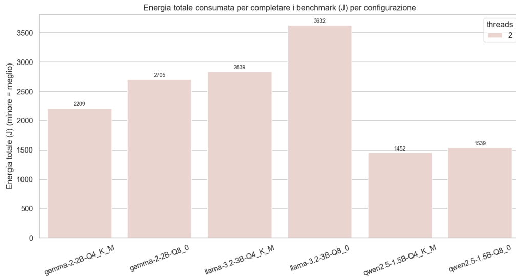
Figura 4.2: Energia totale consumata da ciascuna configurazione per completare la suite di benchmark.
