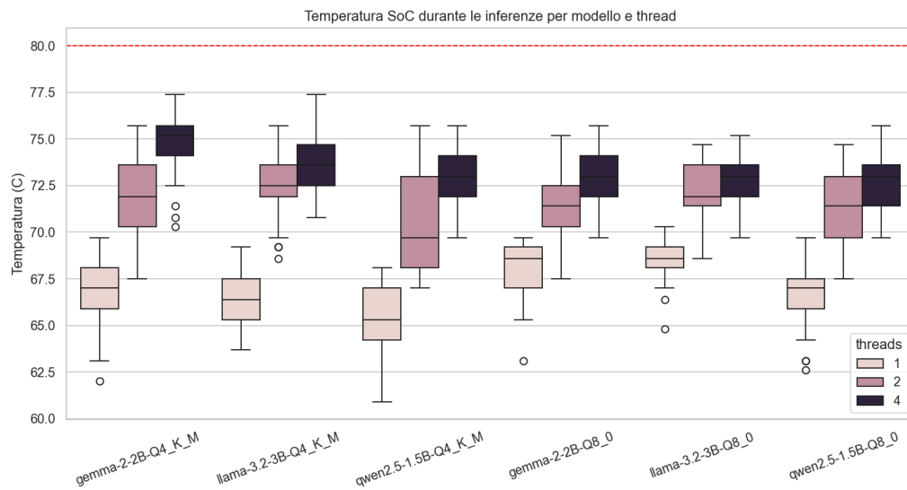
Figura 4.11: Distribuzione della temperatura del SoC durante le inferenze.
