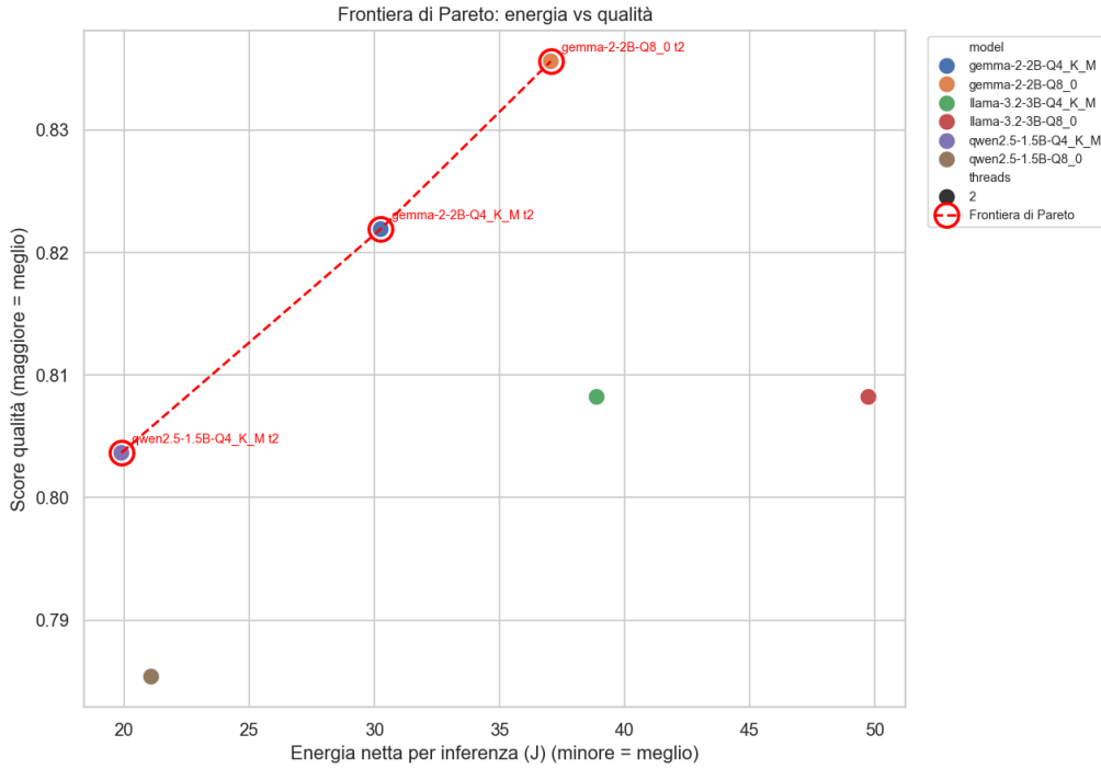
Figura 4.6: Frontiera di Pareto nel piano energia–qualità (cerchiate in rosso le configurazioni non dominate).
