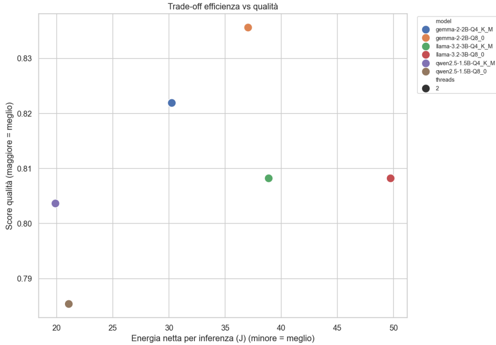
Figura 4.5: Compromesso tra efficienza energetica e qualità delle risposte.
