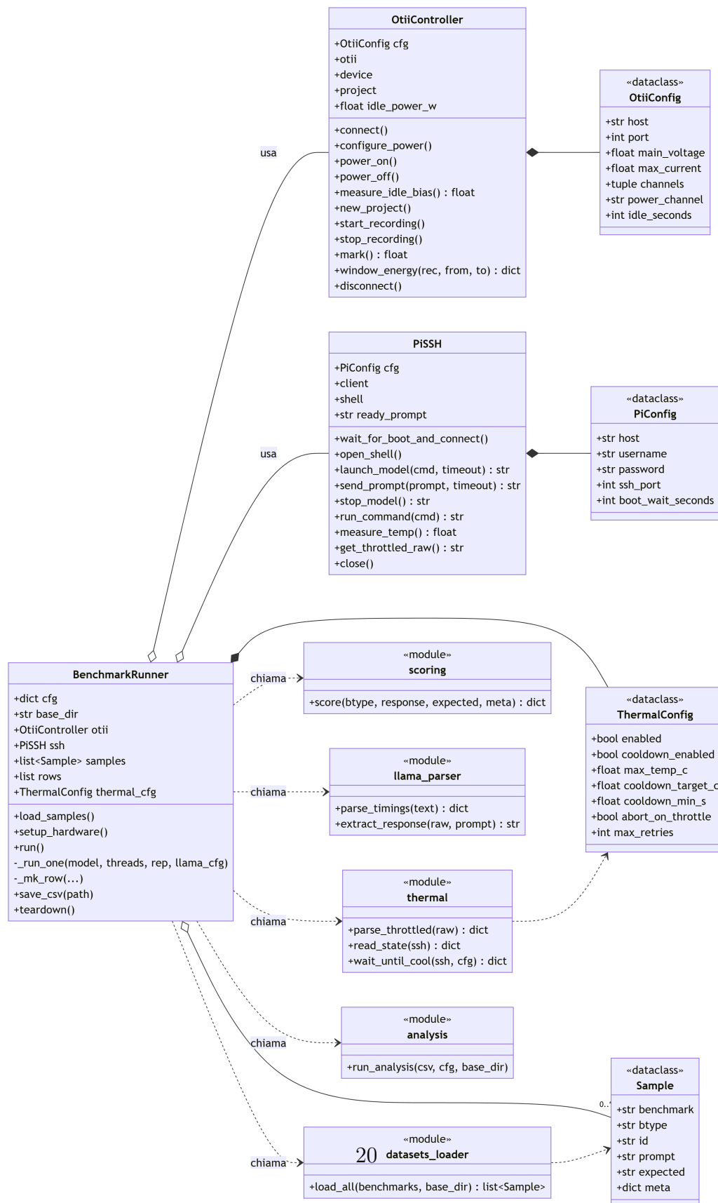
Figura 3.1: Diagramma delle classi dello script di automazione.
